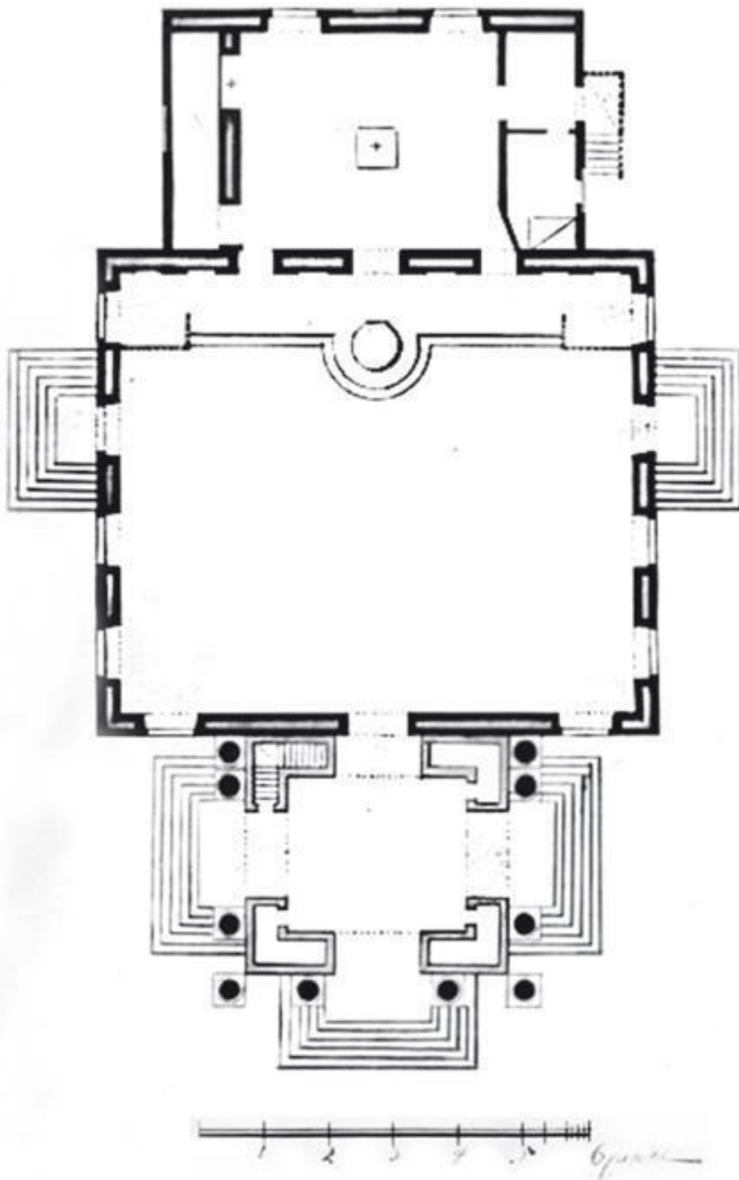
План Троицкого собора, построенного в 1756 г.
