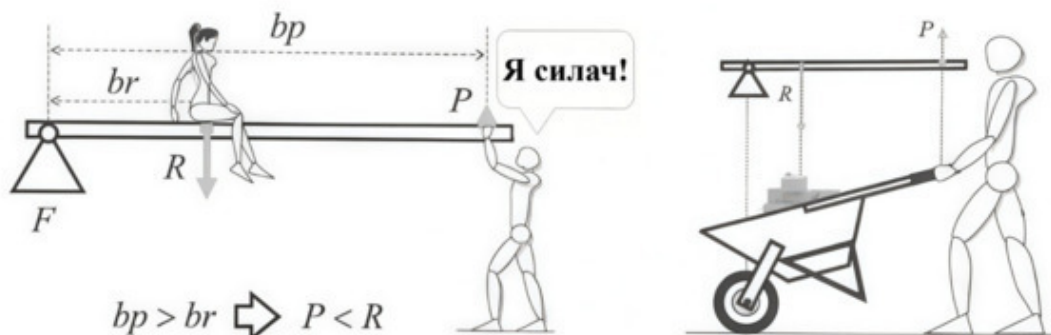
Рисунок 2.39. Рычаг второго рода. Всегда выгодный. Встречается в природе так же редко, как и тишина в зоне кроссфита
