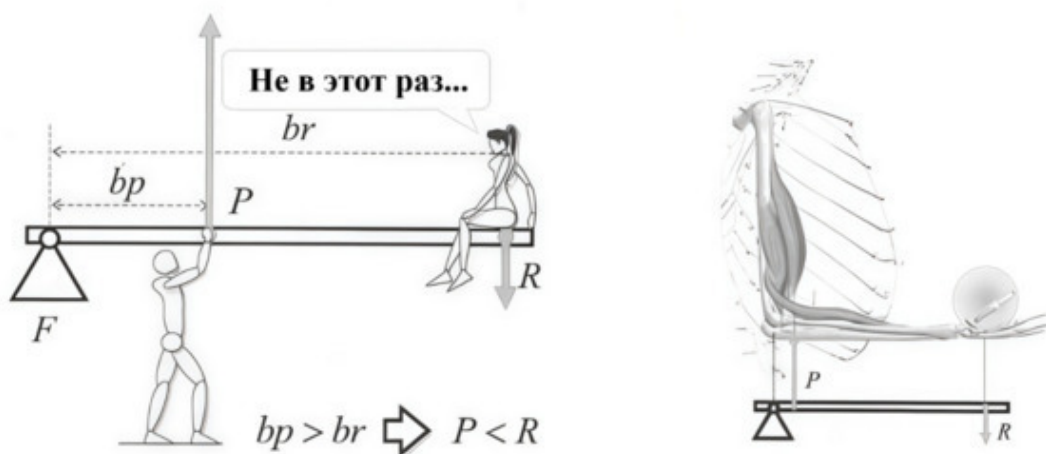
Рисунок 2.40. Рычаг третьего рода. Всегда невыгодный. Знакомьтесь, это про вас и ваш бицепс
