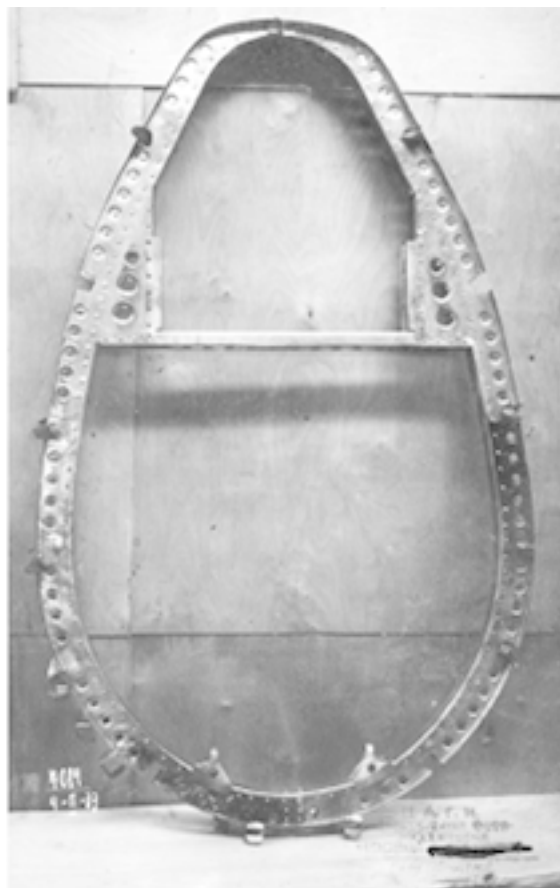
3-й шпангоут с узлами крепления лонжеронов центроплана
