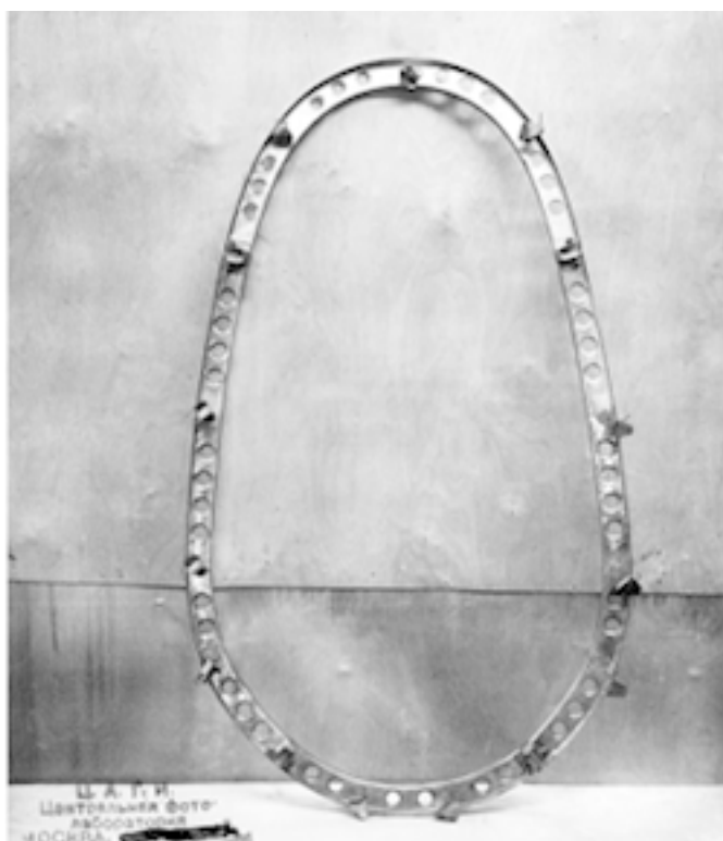
5-й шпангоут фюзеляжа
