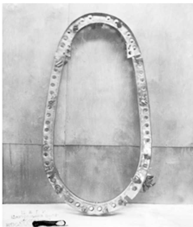
7-й шпангоут фюзеляжа И-14
