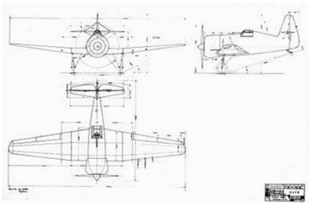
Чертеж общего вида истребителя АИТ-31
