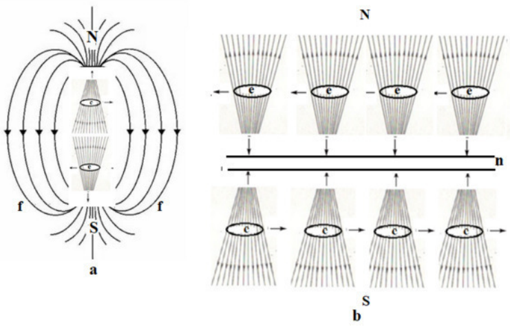
Рис.2 Схема магнитного поля вокруг постоянного магнита
