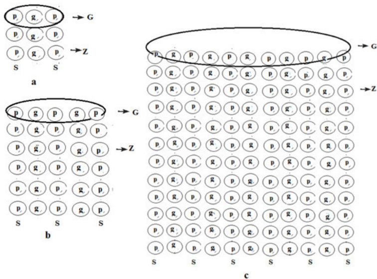
Рис.2. Схема изображения различных видов черных дыр. а – микроскопических; б – образованные в результате коллапса массивных звезд; с – сверхмассивные; S – силовая нить; p – протон; g – гравитон
