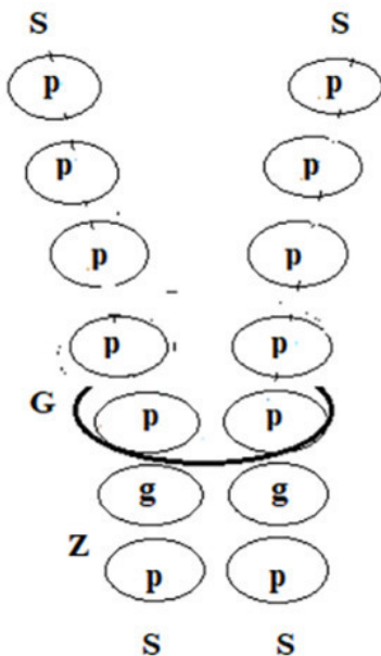
Рис. 1 Схема формирования структуры черной дыры
