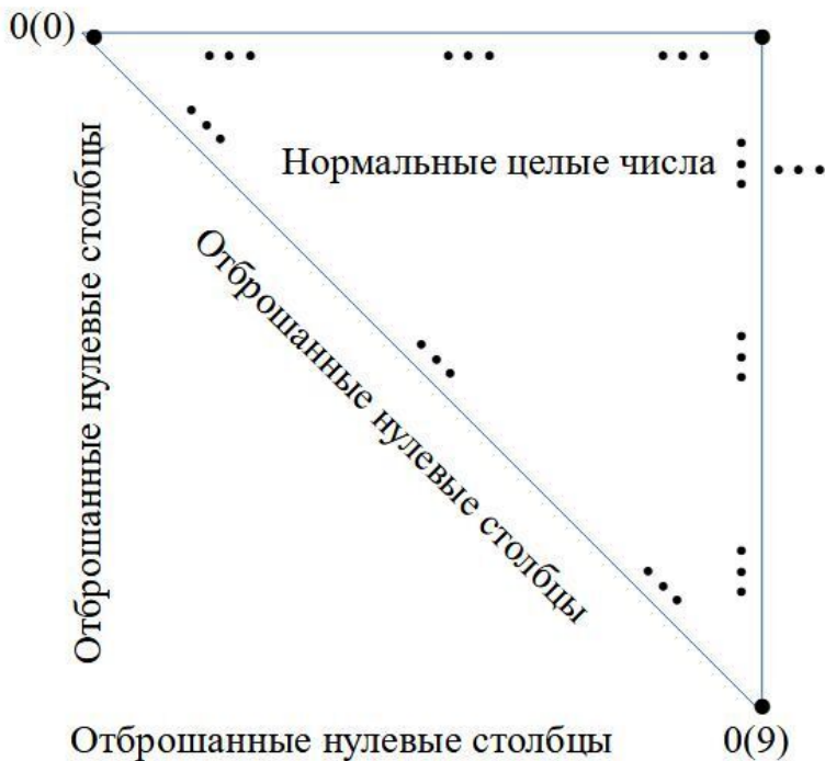
Рисунок 7 Форма массива нормальных целых чисел
