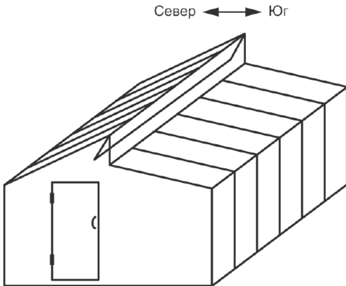
Теплица Митлайдера
