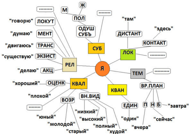
Рис. 3. Самоидентификация Я-субъекта
