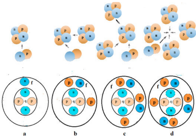
Рис. 5. Предполагаемая схема образования ядер нечетных химических элементов: а – лития; б – бора; с – азота; d – фтора
