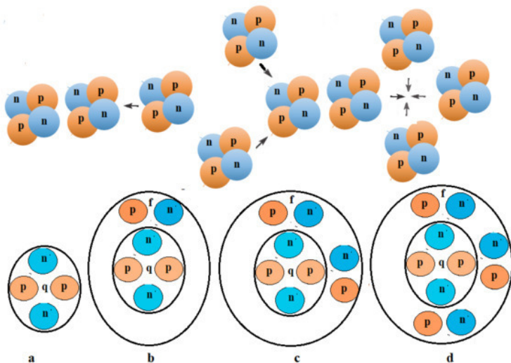
Рис. 3. Предполагаемая схема образования ядер четных химических элементов путем слияния ядер гелия: а – ядро
