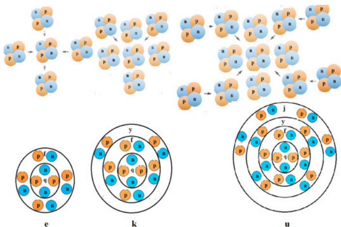
Рис. 4. Предполагаемая схема образования ядер четных химических элементов путем слияния ядер гелия: e – неона; k – кремния; u – железа
