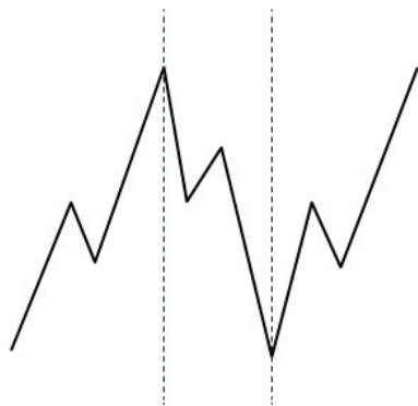
Рисунок 3.8. «Разделение» на составные волны
