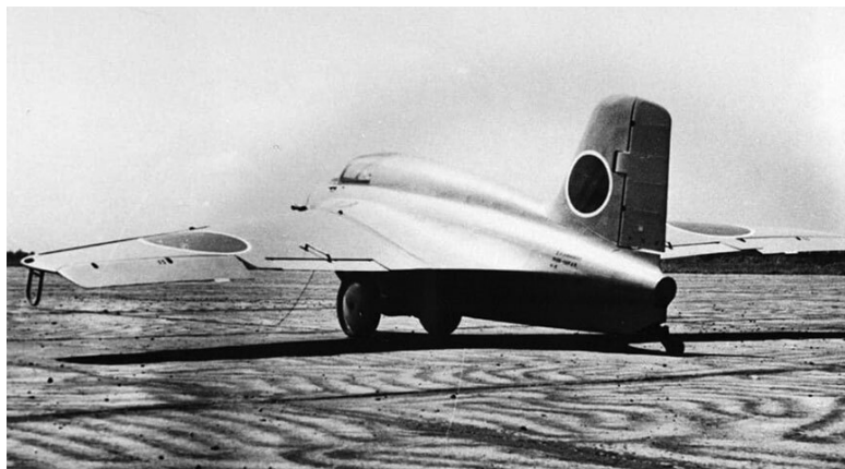
Реактивный БПЛА, построенный в 1945 году в рамках проекта Сюсуй
