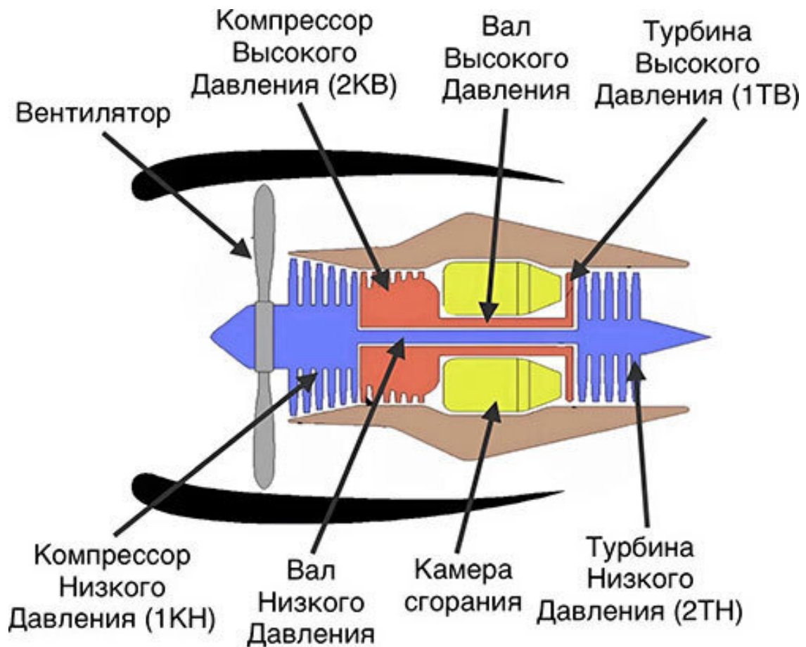
Строение двигателя CFM56-7B
