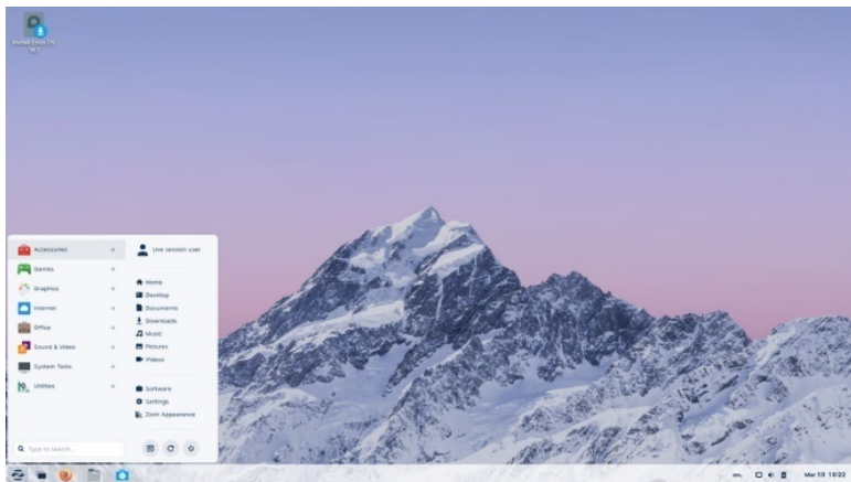
Рисунок 2 Zorin OS
