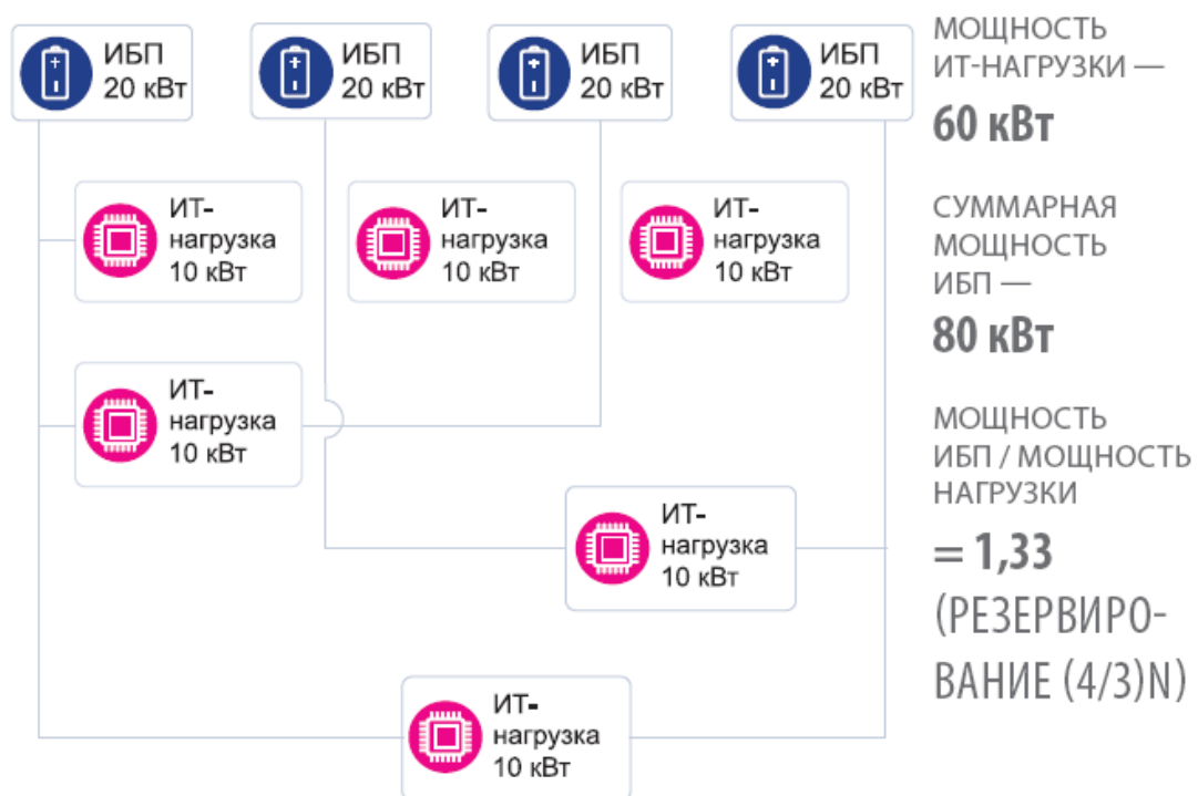
Рис. 5. Резервирование (4/3) N
