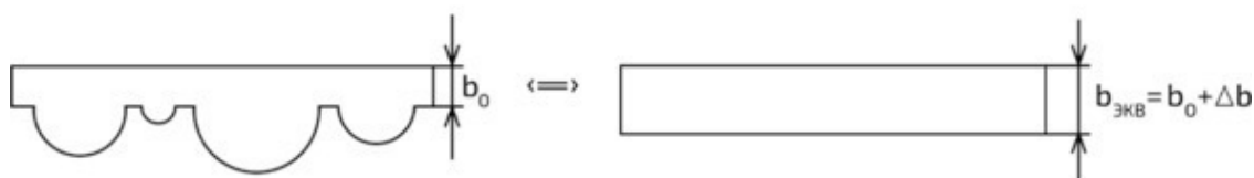
Рисунок 16. Увеличение эквивалентной толщины слоя герметика на \Delta b из-за заполнения герметиком открытых пор пены
