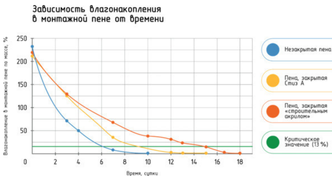
Рисунок 24. Зависимость влагосодержания в монтажной пене от времени
