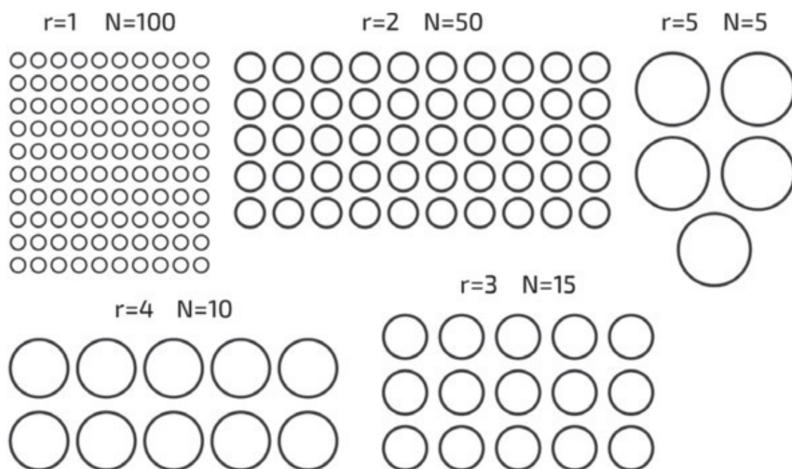
Рисунок 18. Заготовка макета с использованными в расчете геометрическими размерами. Радиус 0,5 мм не использован
