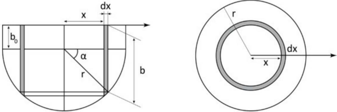
Рисунок 17. Схема расчета потока пара через фрагмент слоя герметика с выпуклостью в области расположения поры
