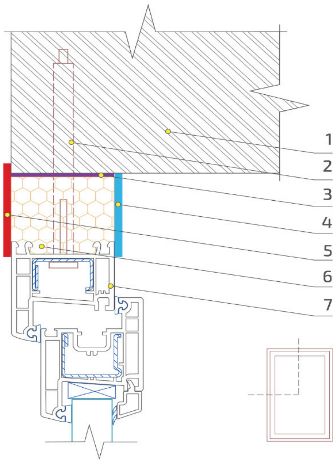
Рисунок 11. Схема монтажного шва узла примыкания оконного блока к стеновому проему без четверти (1 – кирпичная стена; 2 – анкерный дюбель; 3 – дополнительный слой монтажного шва; 4 – пароизоляция монтажного шва; 5 – гидроизоляция монтажного шва; 6 – пена монтажная; 7 – оконный блок)
