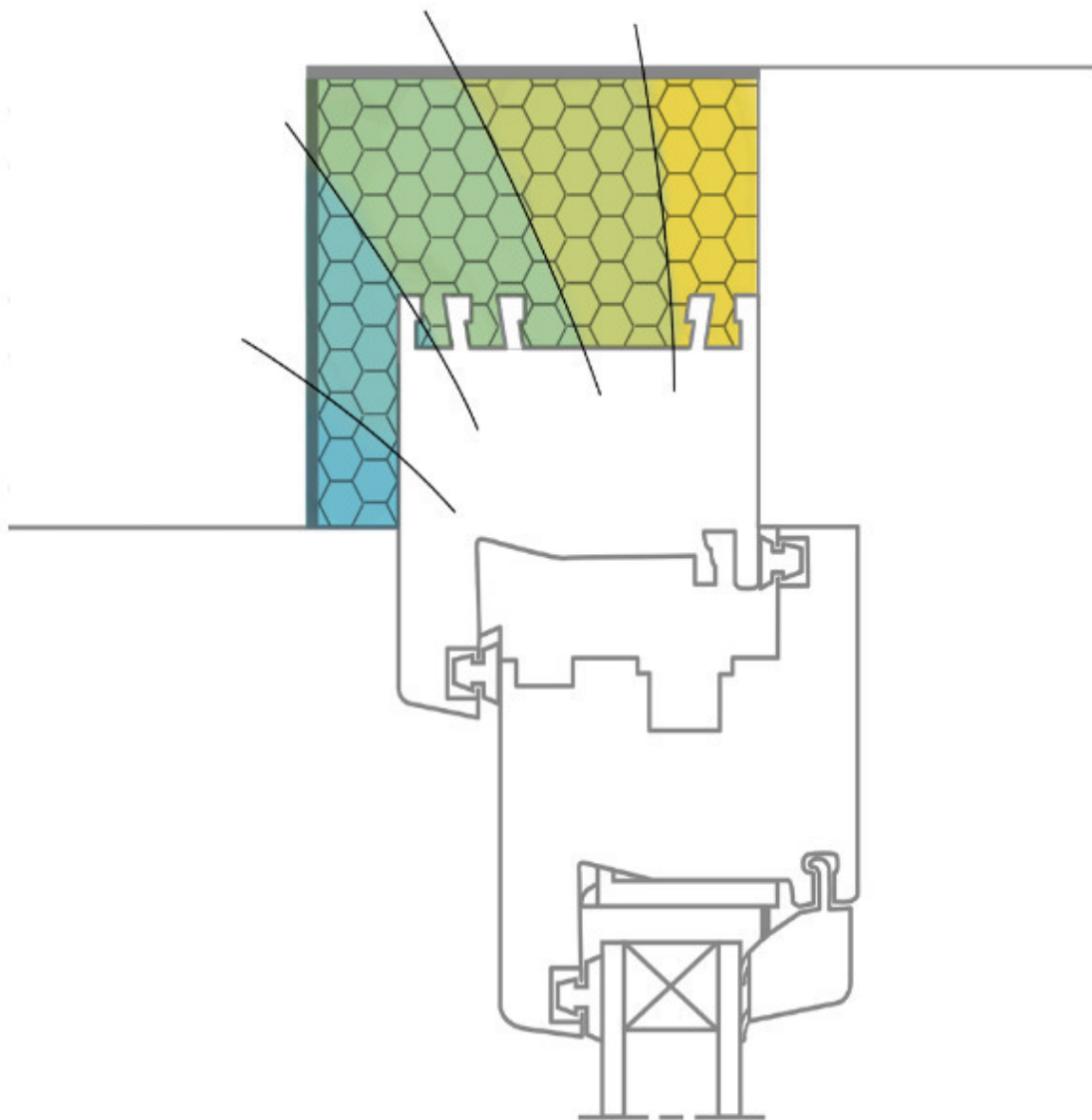
Рисунок 2. Распределение изотерм в монтажном шве до образования трещины
