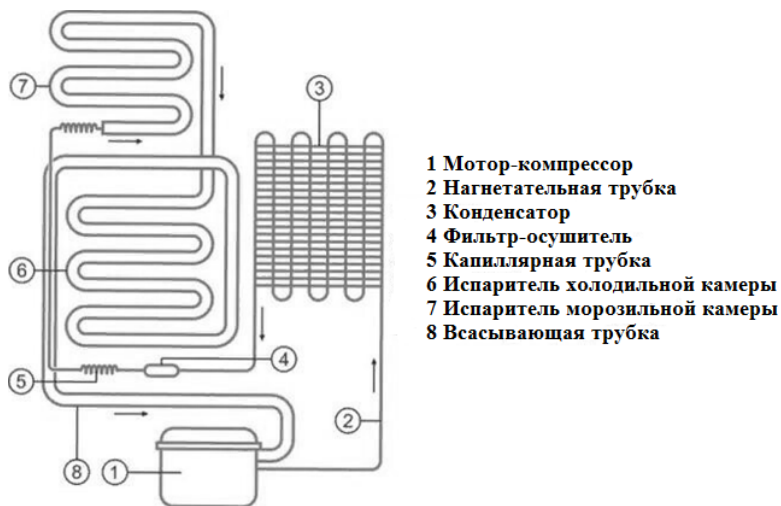
Рис. 1. Устройство парокомпрессионной холодильной машины
