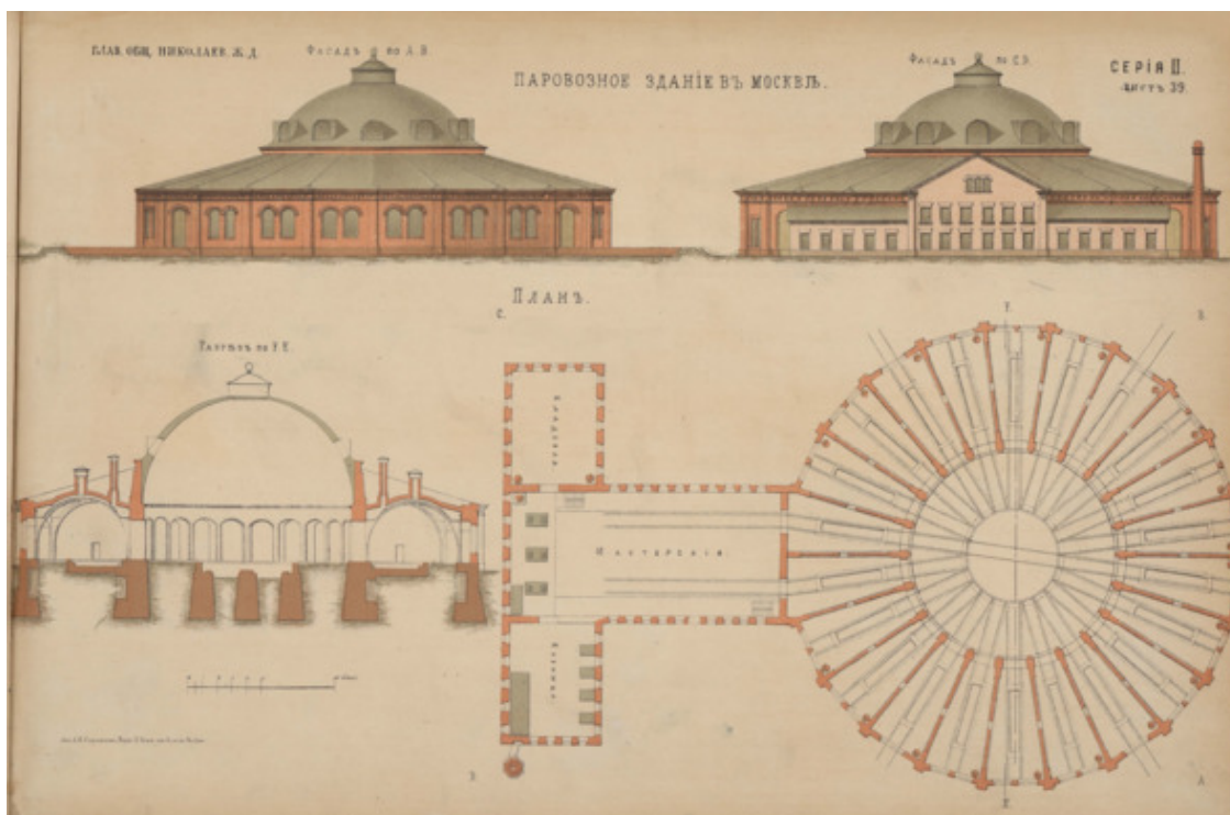
Паровозное здание в Москве. Альбом чертежей сооружений Российских железных дорог, 1872 г.
