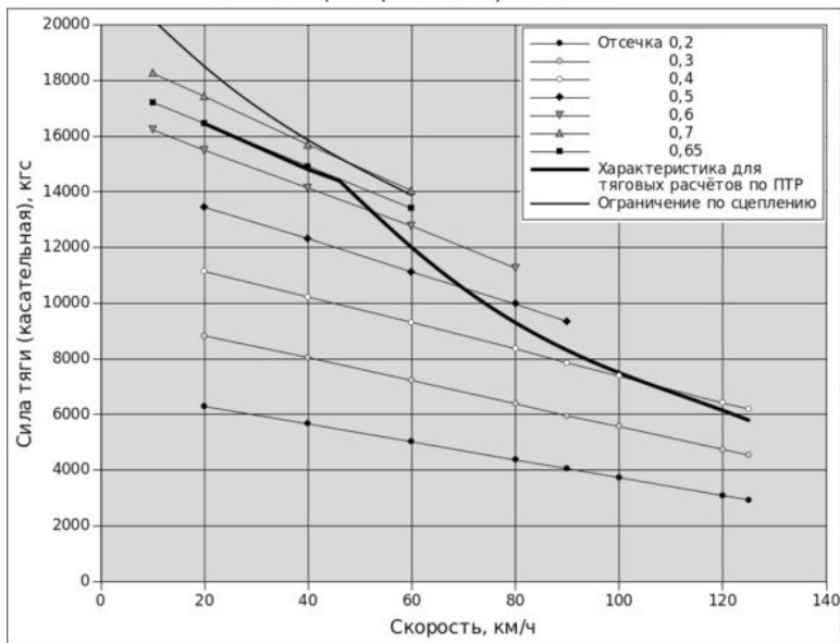
Тяговые характеристики паровоза ПЗ6
