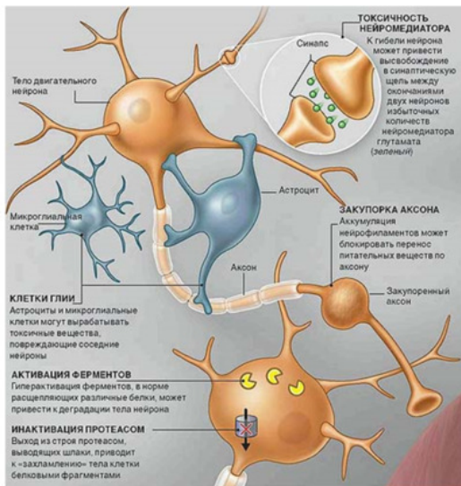
Рис. 1. Установленные негенетические молекулярно-биологические механизмы развития бокового амиотрофического склероза
