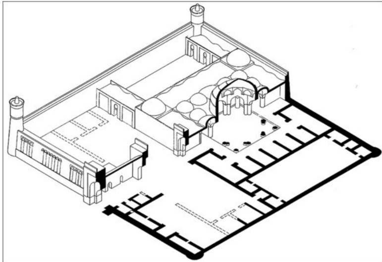
Рис. 21. Рабат-и Малик, реконструкция 2-го периода. XII в.
