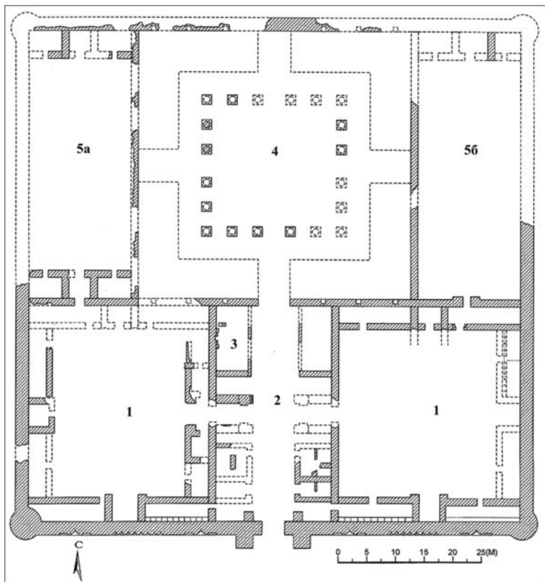
Рис. 14. Рабат-и Малик (перс. «Царская крепость»), план
