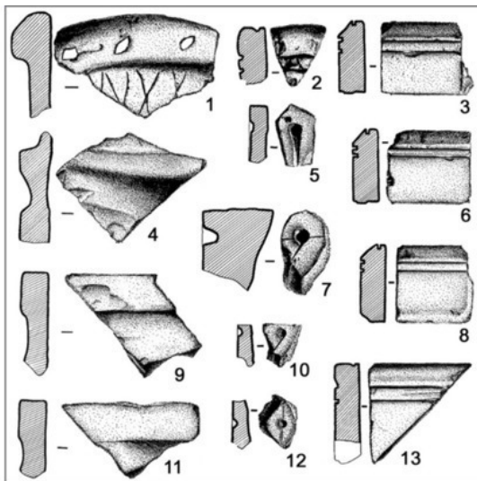
Рис. 20. Фрагменты архитектурного декора, неполивные изразцы, гравированный ганч. XI — XII вв.
