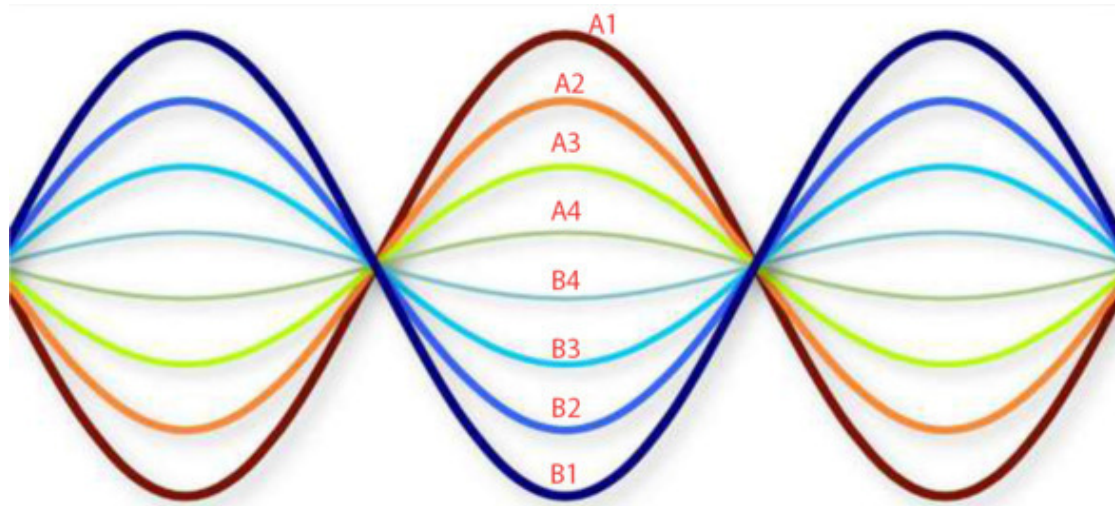
Рис. 33. Стоячие волны
