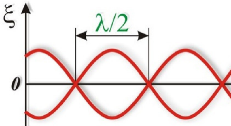
Рис. 32. Стоячая волна
