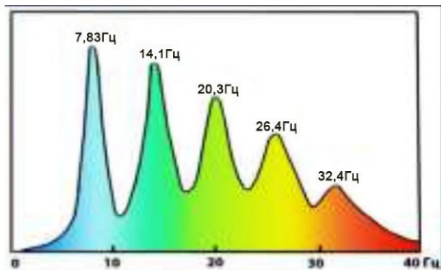
Рис. 20. Резонансы Шумана
