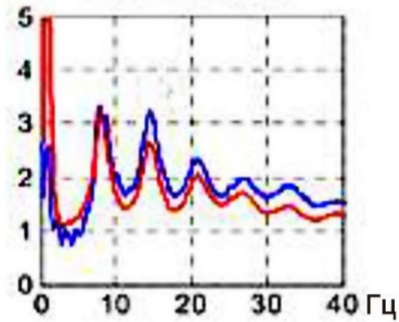
Рис. 21. Сейсмический сигнал, совпадающий с резонансами Шумана
