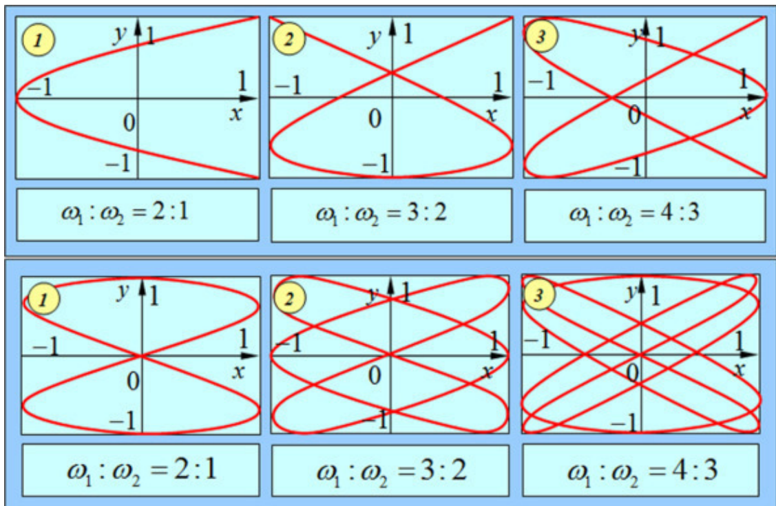
Рис. 47. Фигуры Лиссажу
