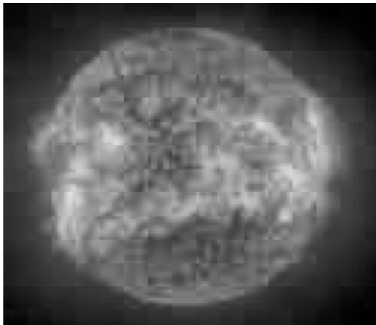
Figura 1.4.- Manchas solares
