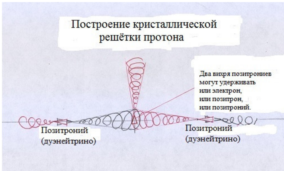
Рис.5 Взаимодействие двух позитрониев в кристаллической решётке протона
