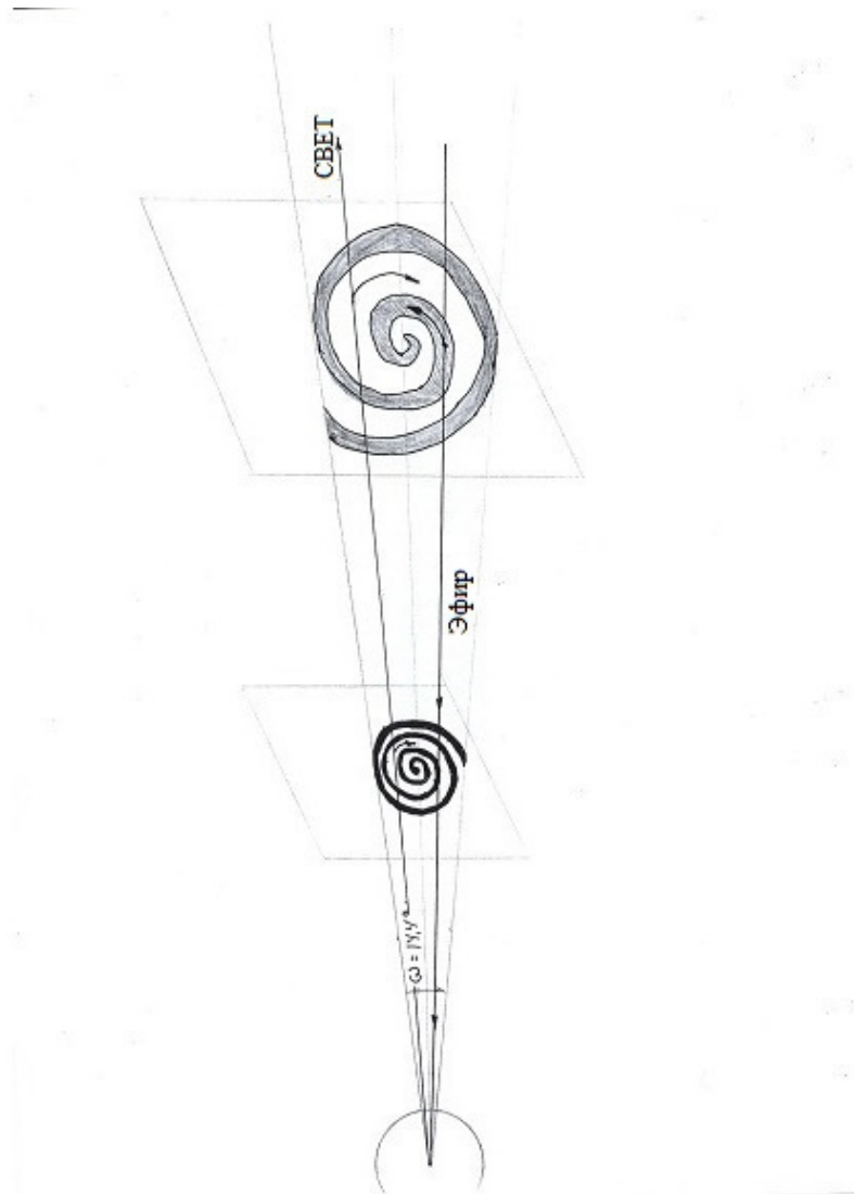
Рис.24 СВЕТОЭфирный поток
