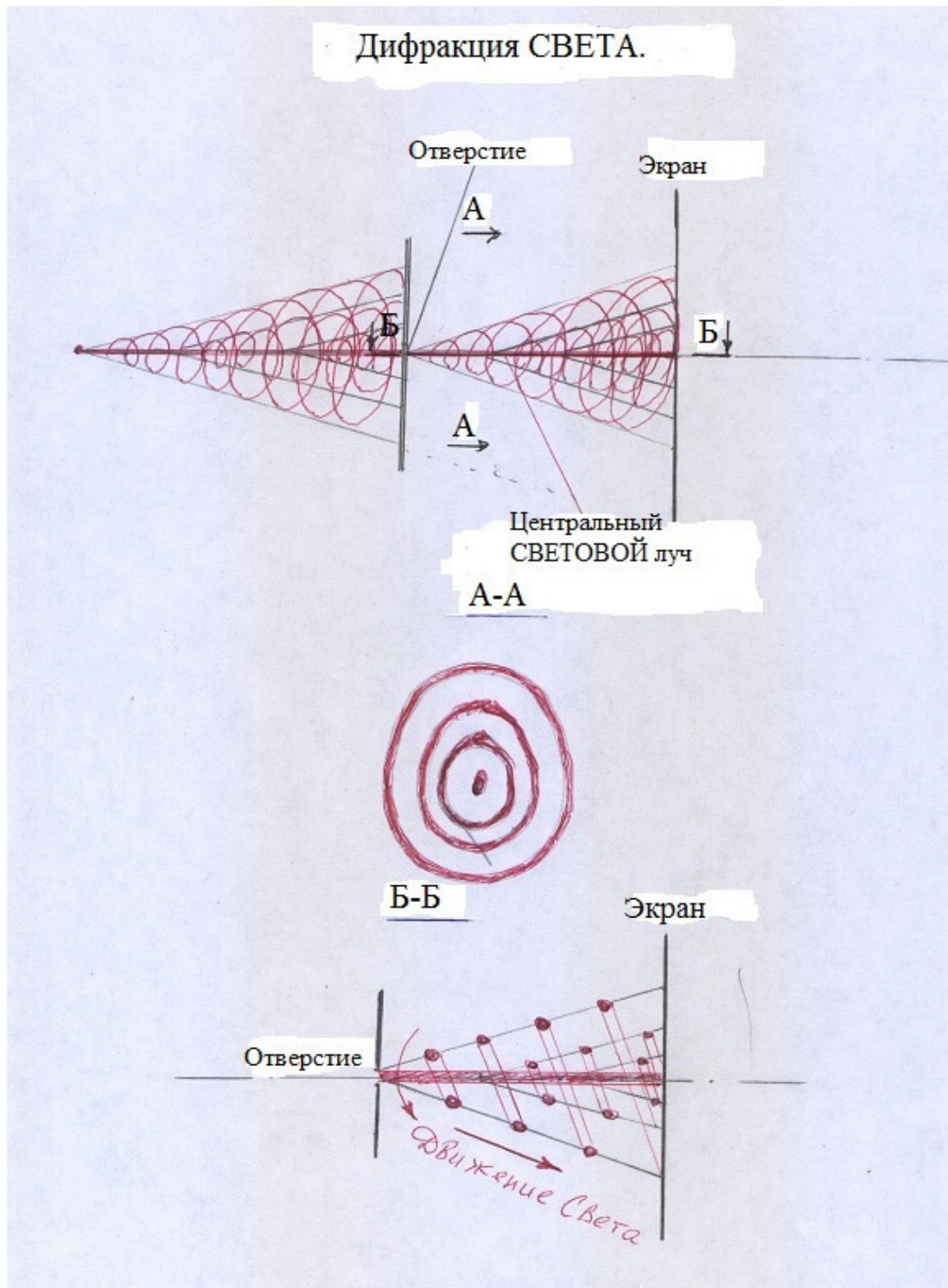
Рис.32 Дифракция СВЕТА
