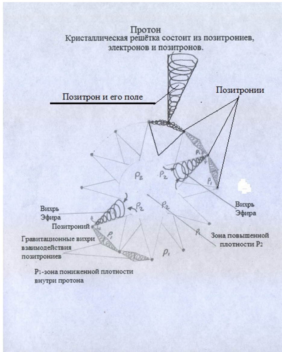
Рис. 6 Протон
