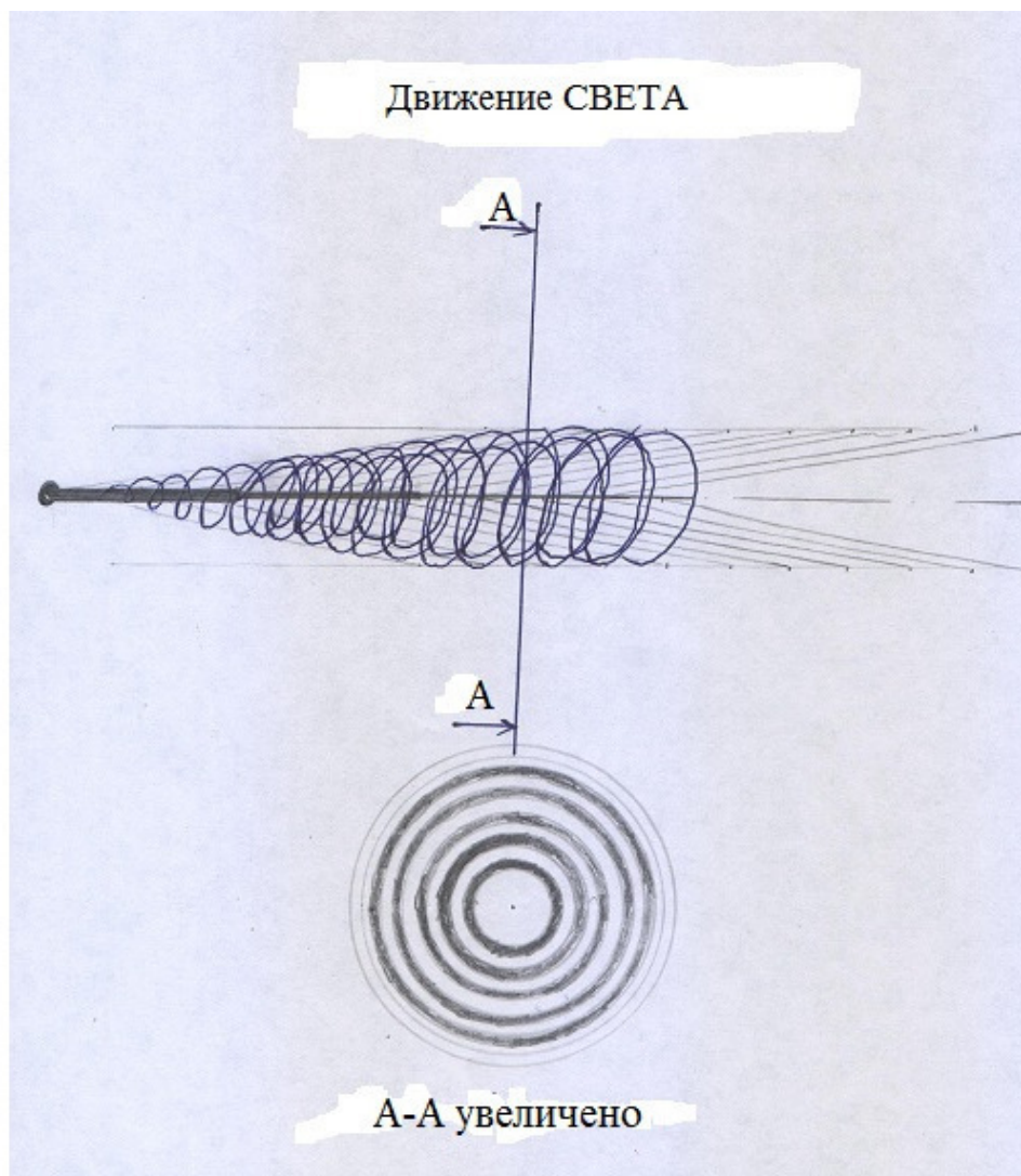
Рис.31 СВЕТОЭфирный поток
