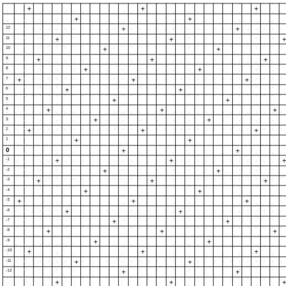
Квинто-полутоновая схема
