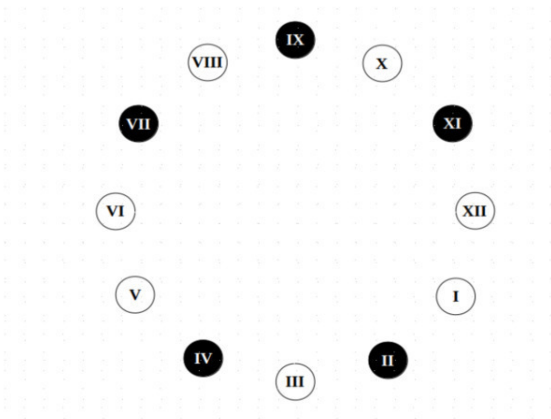
Полутоновый круг
