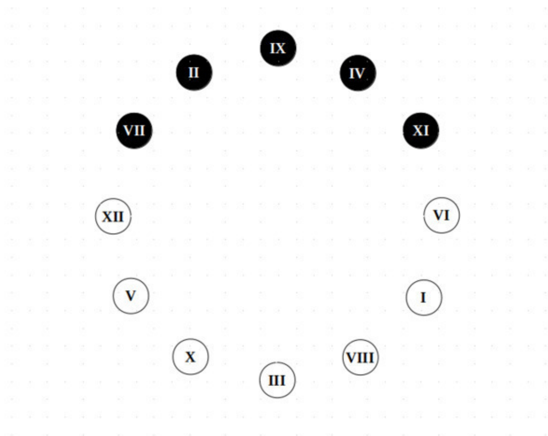
Квинтовый круг
