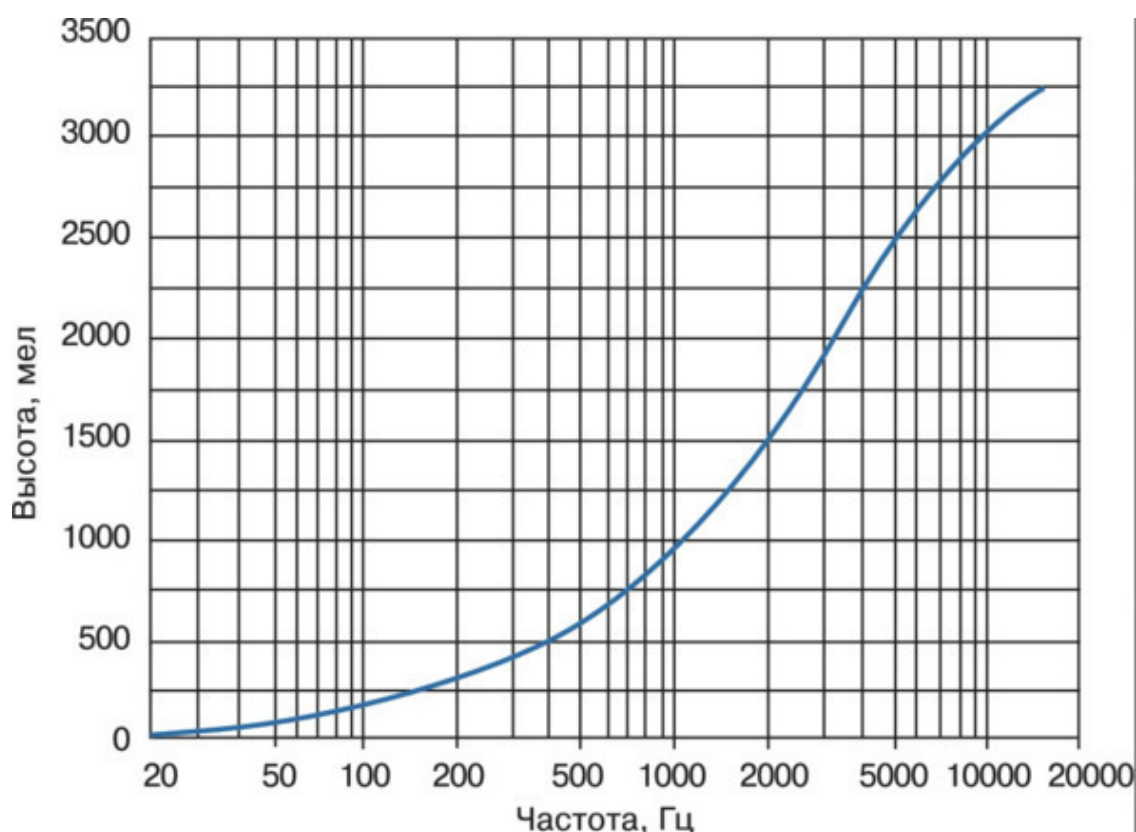
Шкала частот
