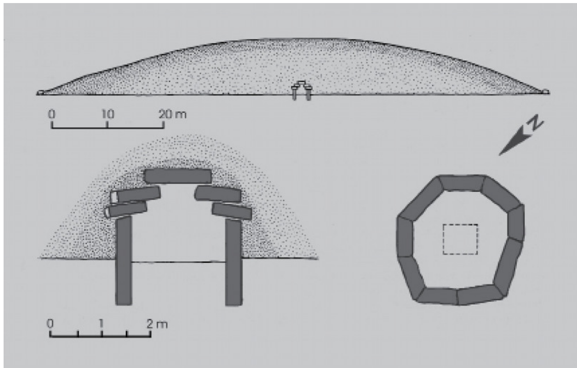
Abb. 6 Seddin, Königsgrab. Zeichnerische Rekonstruktion (Schnitt durch den Grabhügel und Grundriss der Grabkammer).
