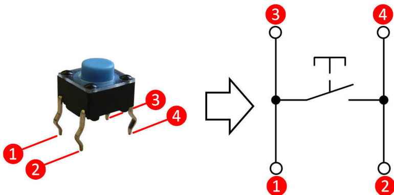
Abb. 5: Der Mikrotaster
