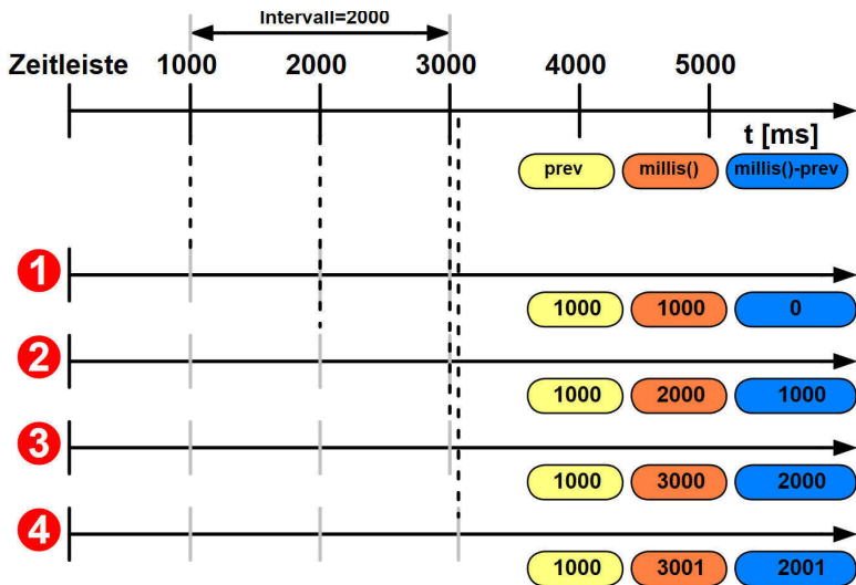
Abb. 5: Der zeitliche Verlauf der Intervallsteuerung
