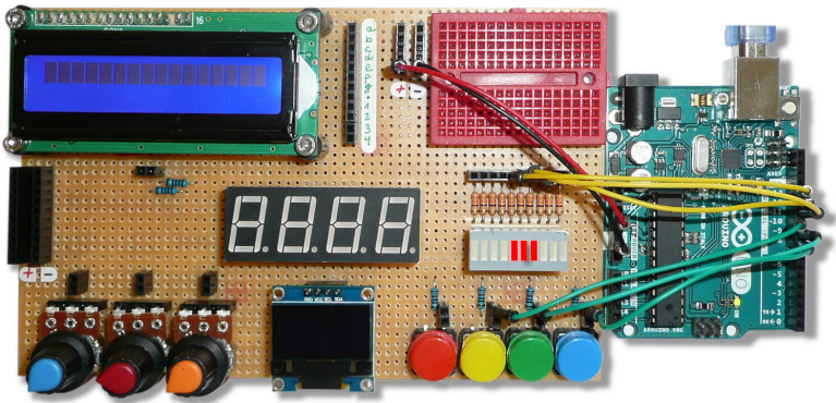
Abb. 11: Der Versuchsaufbau mit zusätzlichen Tastern
