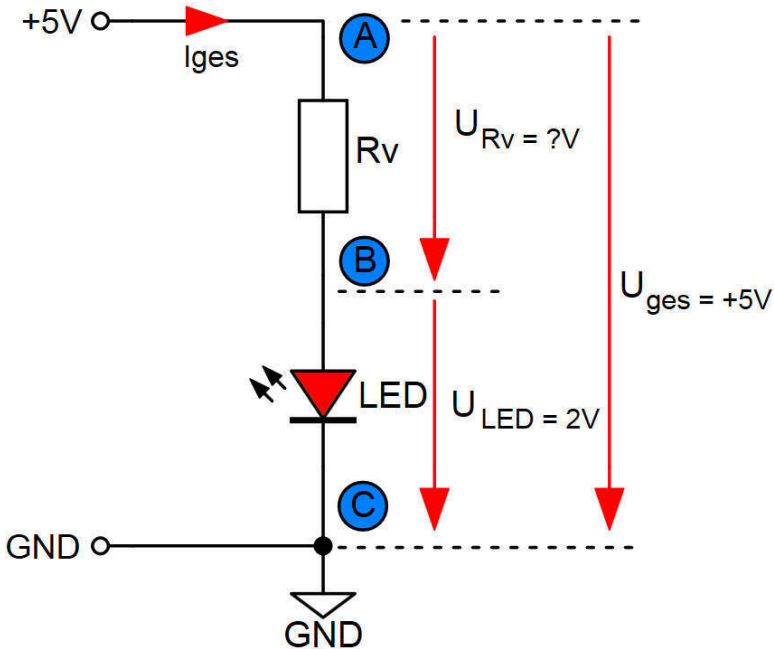
Abb. 5: Eine LED mit Widerstand
