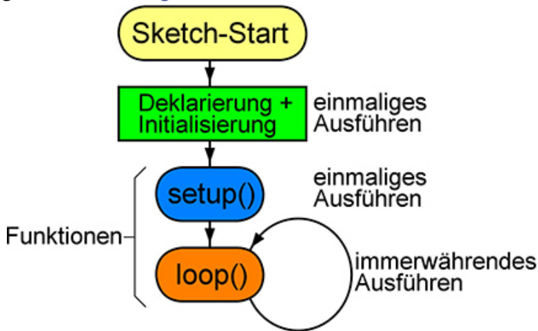
Abb. 3: Die grundlegende Struktur eines Sketches
