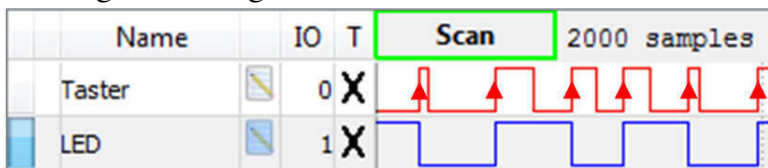
Abb. 6: Das Toggeln der LED durch den Taster
