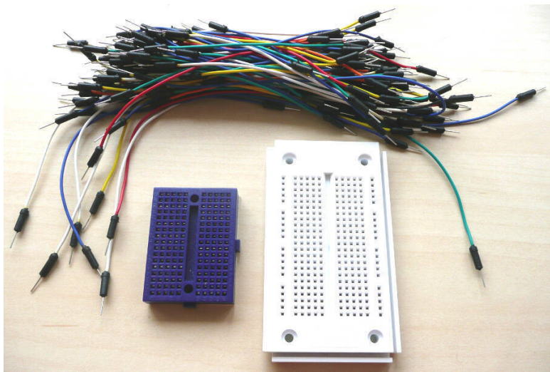
Abb. 19: Verschiedene Breadboards und flexible Steckbrücken
