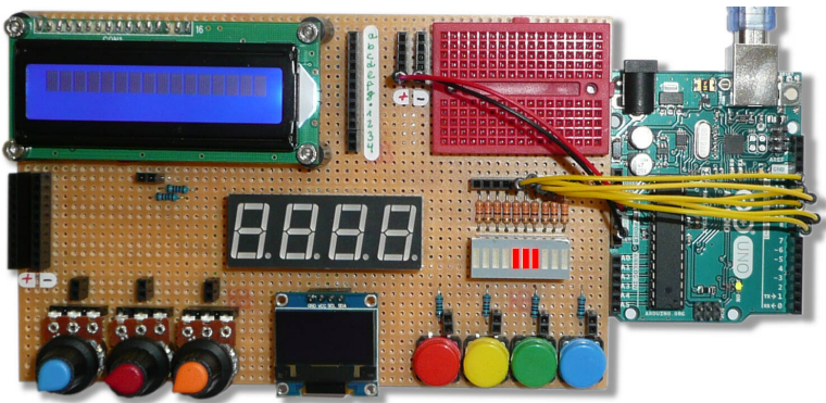
Abb. 6: Der Versuchsaufbau mit sechs Leuchtdioden auf dem Arduino Discoveryboard
