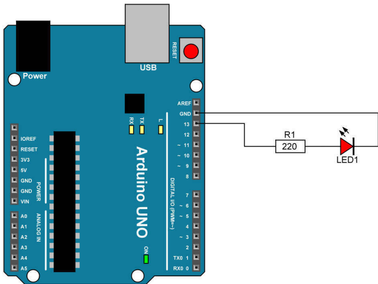
Abb. 1: Der Schaltplan
