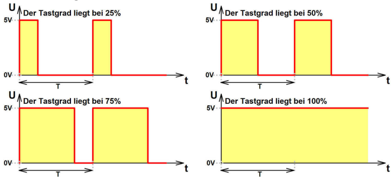
Abb. 16: Einige PWM-Beispiele
