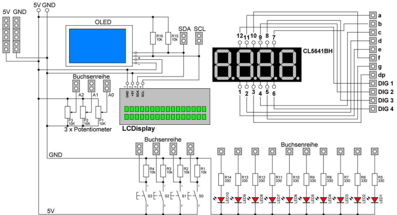
Abb. 2: Der Discoveryboard-Schaltplan
