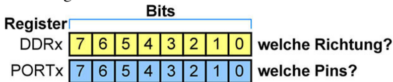
Abb. 3: Die Register DDR x und PORT x
