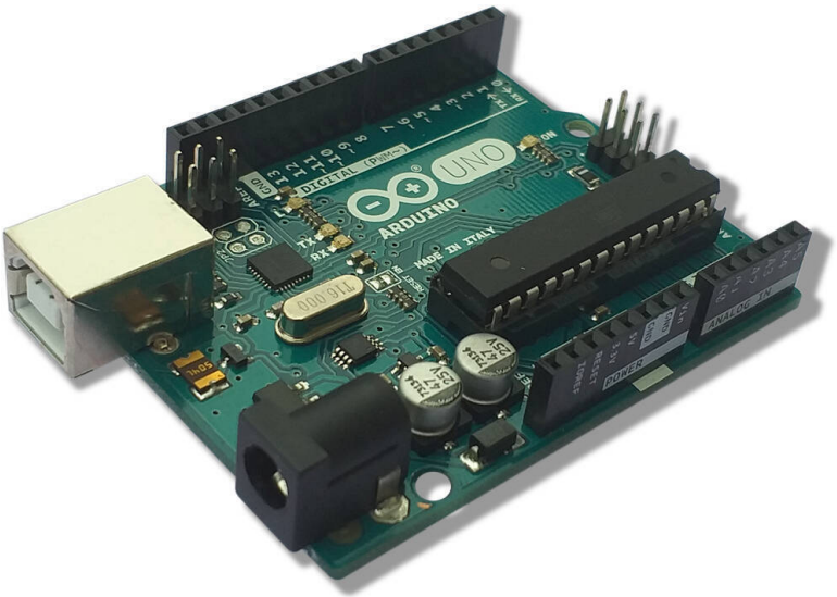
Abb. 1: Der Arduino Uno – das Original
