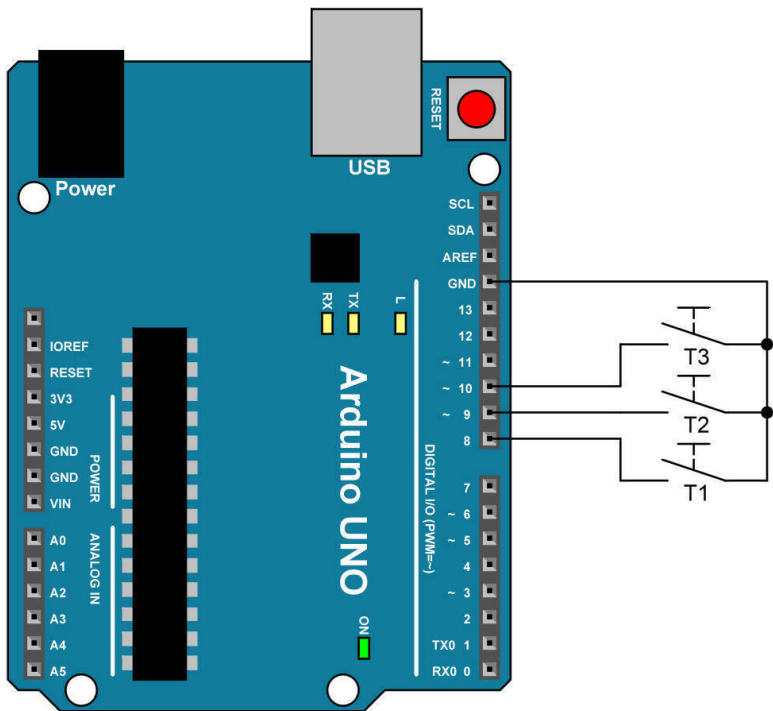
Abb. 16: Eine Schaltung mit drei Tastern
