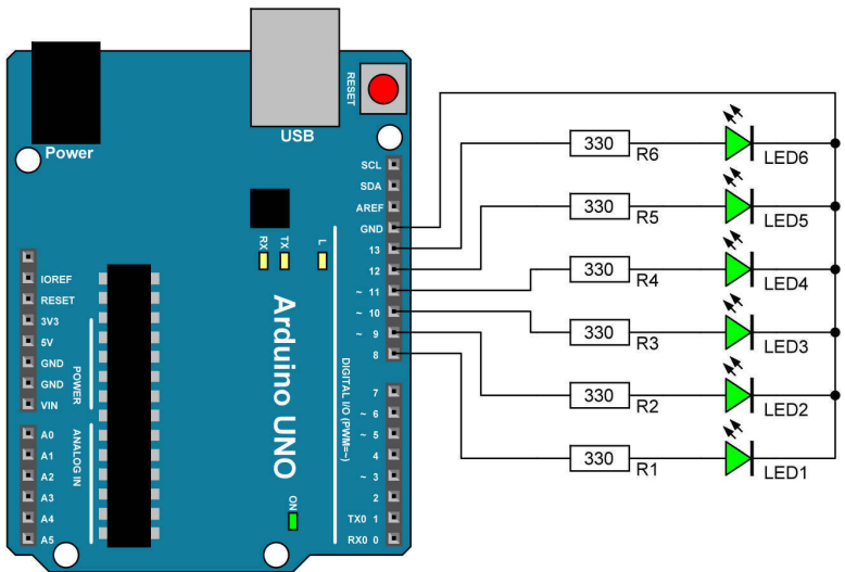
Abb. 5: Der Schaltplan mit 6 LEDs
