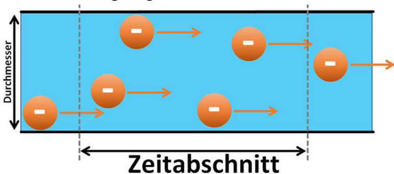
Abb. 9: Wenige Elektronen auf dem Weg durch einen Leiter
