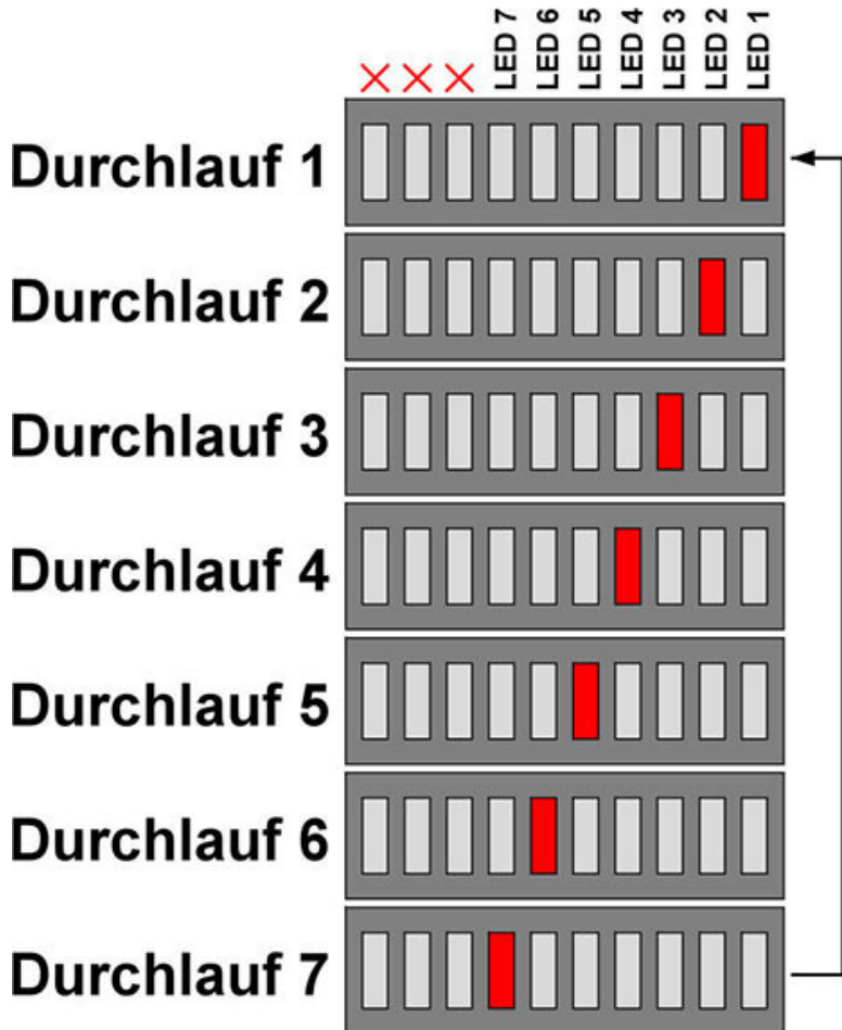
Abb. 1: Die Leuchtsequenz der sieben LEDs
