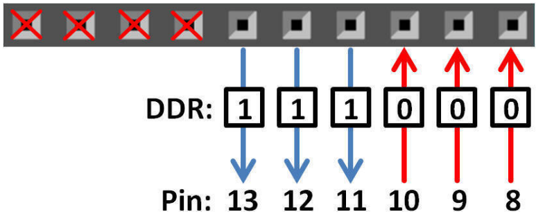
Abb. 4: Die Konfiguration von Port B
