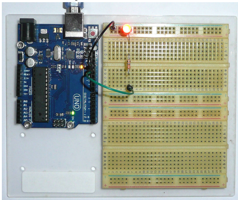
Abb. 2: Der Schaltungsaufbau auf einem kleinen Arduino-
