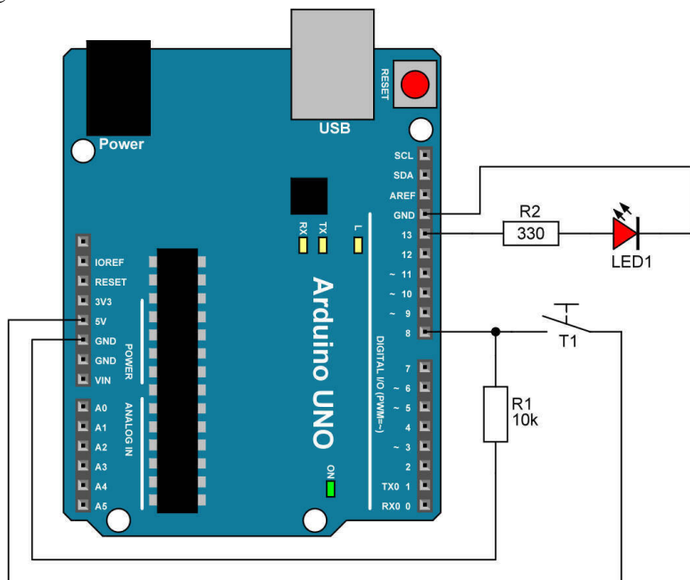
Abb. 6: Der Schaltplan zur Tasterabfrage
