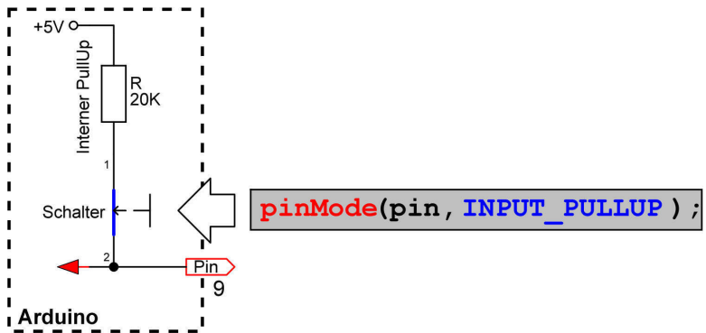
Abb. 3: Der interne Pullup-Widerstand wurde aktiviert
