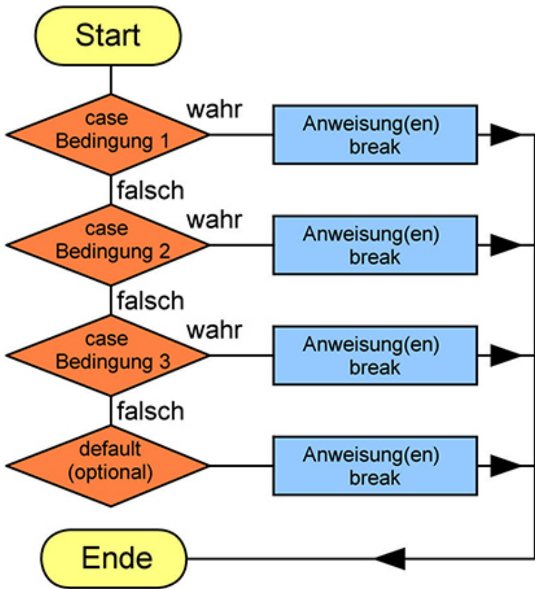
Abb. 5: Das Flussdiagramm einer switch-case-Kontrollstruktur
