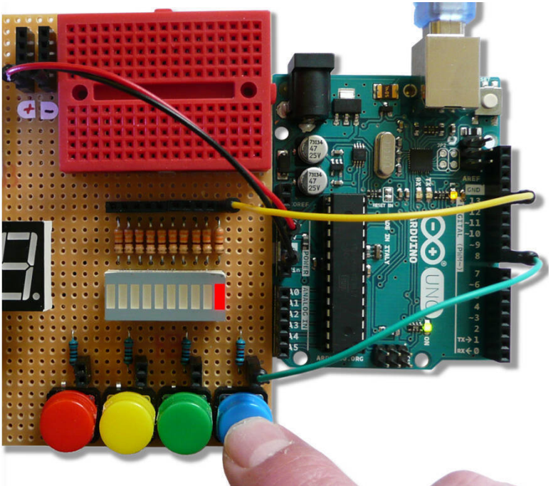
Abb. 7: Der Schaltungsaufbau zur Tasterabfrage auf dem Arduino Discoveryboard
