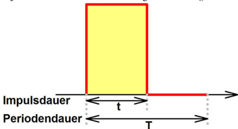
Abb. 15: Impuls- und Periodendauer im zeitlichen Verlauf
