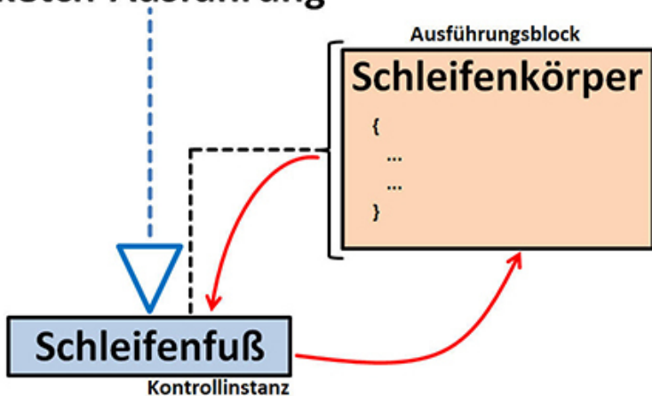
Abb. 9: Grundsätzlicher Aufbau einer fußgesteuerten Schleife
