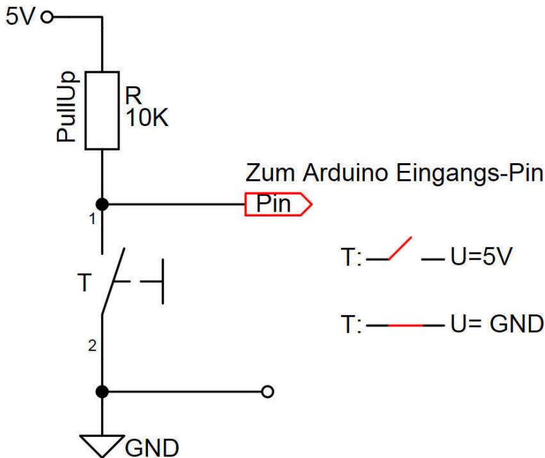
Abb. 15: Ein offener Eingang mit Pullup-Widerstand
