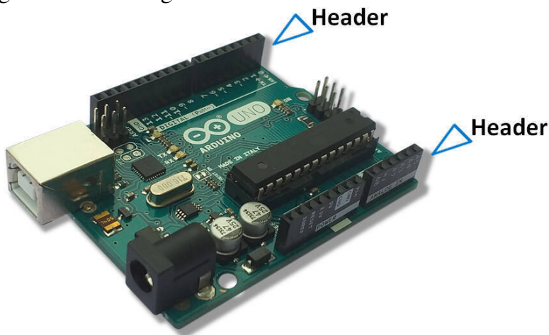
Abb. 10: Die Header des Arduino Uno
