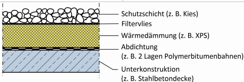
Bild 7: Beispielquerschnitt eines Umkehrdaches (Quelle: Schmidt)
