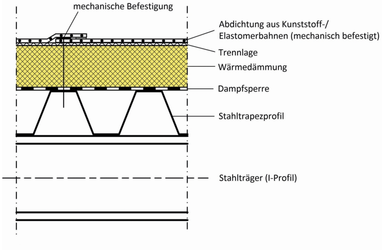
Bild 26: Nicht belüftetes Dach (Quelle: Schmidt)
