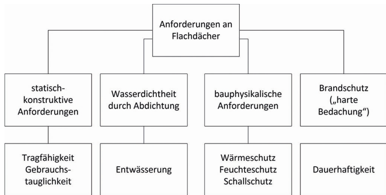
Bild 32: Anforderungen an Flachdächer (Quelle: Schmidt)
