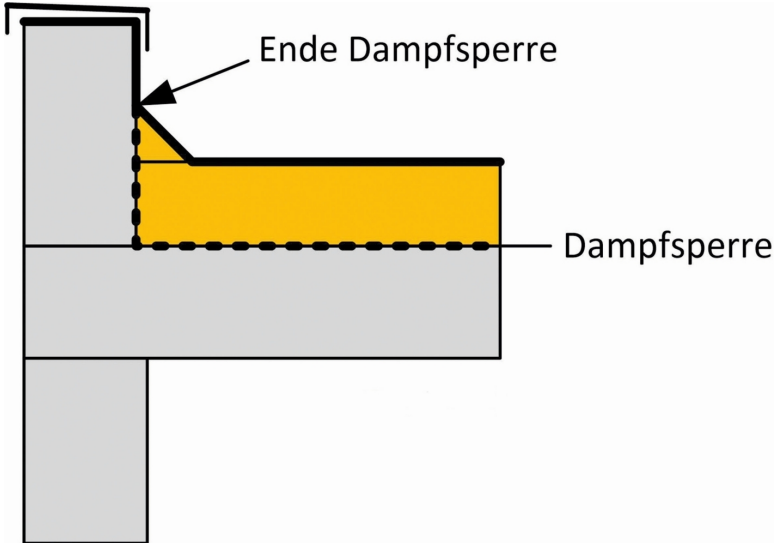
Bild 17: Dampfsperre im Bereich eines Anschlusses (Quelle: Schmidt)
