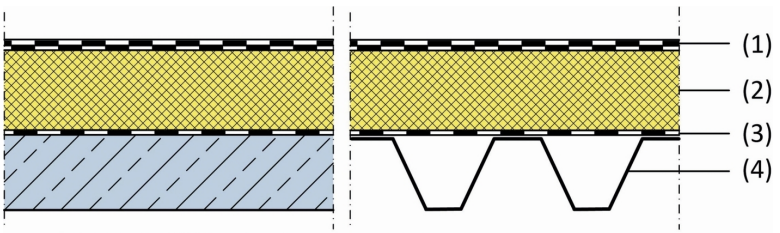
(A) nicht belüftetes Dach auf Stahlbetondecke
