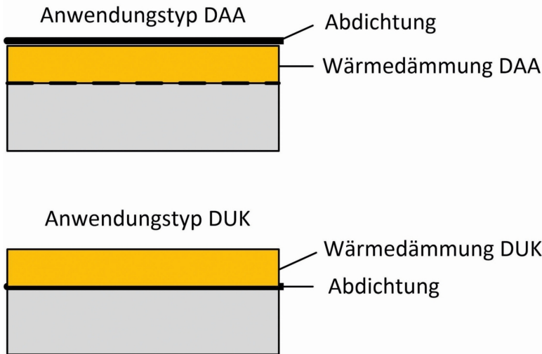
Bild 19: Anwendungstypen DAA und DUK (Quelle: Schmidt)
