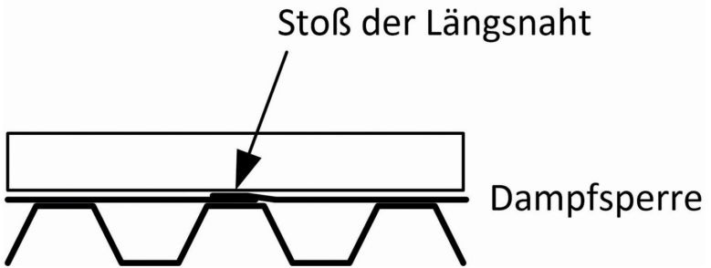
Bild 18: Verlegung einer Dampfsperre auf Stahltrapezprofilen (Quelle: Schmidt)
