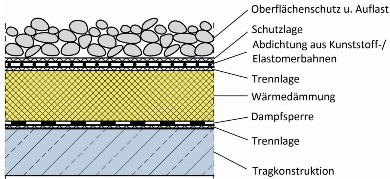
Bild 25: Nicht belüftetes Dach (Quelle: Schmidt)
