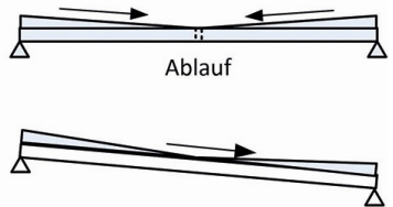
nicht funktionierende Entwässerung
