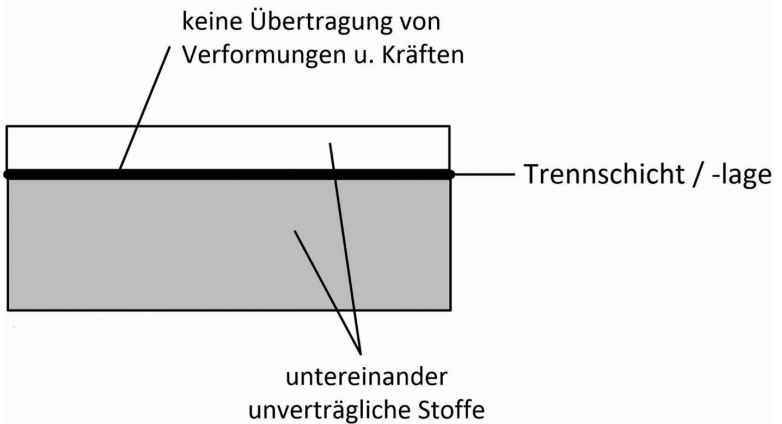
Bild 16: Funktion von Ausgleichs- und Trennschicht/ Trennlage (Quelle: Schmidt)
