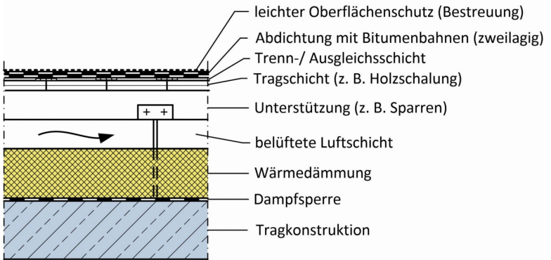
Bild 28: Umkehrdach auf Stahlbetondecke (Quelle: Schmidt)
