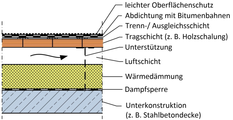
Bild 10: Beispielquerschnitt für ein belüftetes Flachdach (Kaltdach) (Quelle: Schmidt)
