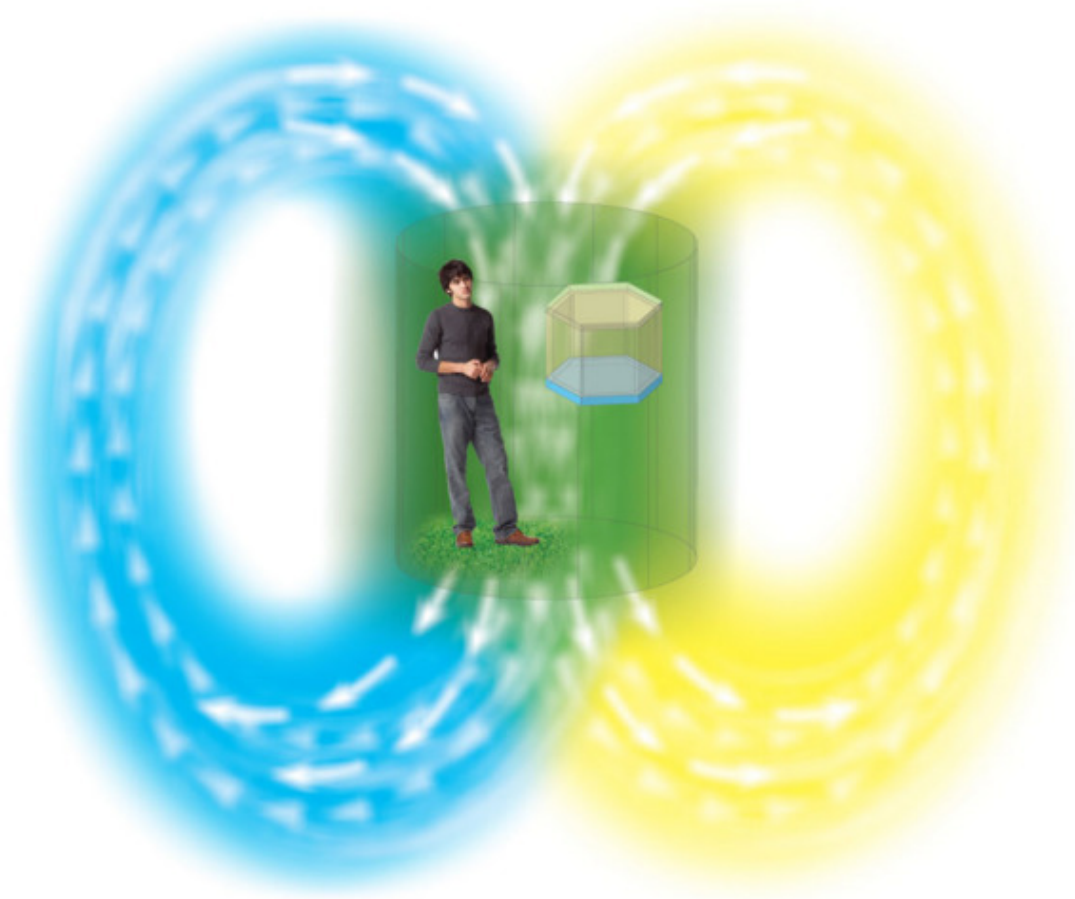
Рис. 10.3. Метод тора.
