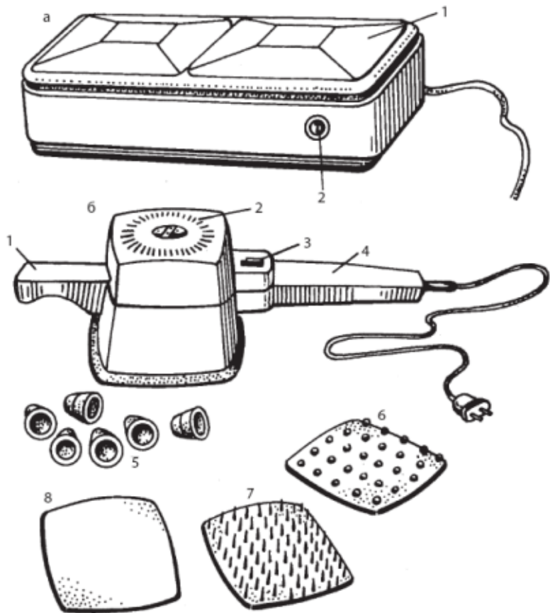
Рис. 2. Массажные аппараты: а – общий вид ПЭМ-1: 1 – вибрирующая площадка; 2 – регулятор частоты вибрации; б – вибромассажер электрический ЭЛВВО: 1 – дополнительная рукоятка; 2 – корпус; 3 – выключатель; 4 – основная
