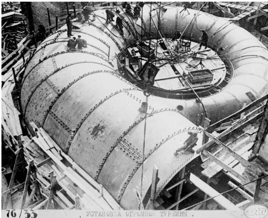
Монтаж турбины на ДнепроГЭС в 1932 г.
