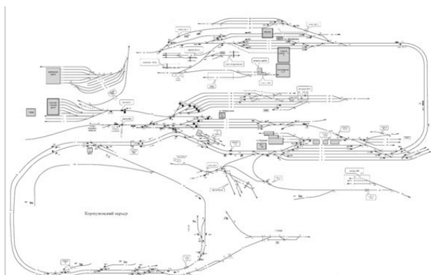
Рис. 2.7. Немасштабная схема путевого развития предприятия
