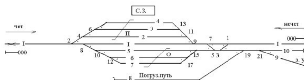
Рис. 2.11. Нумерация путей и стрелок
