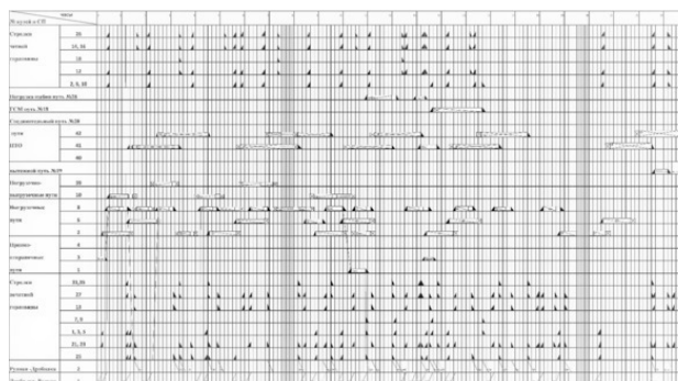
Рис. 2.1. График исполненного движения поездов
