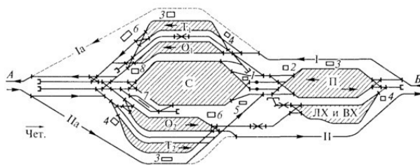
Рис. 2.5. Сортировочная станция
