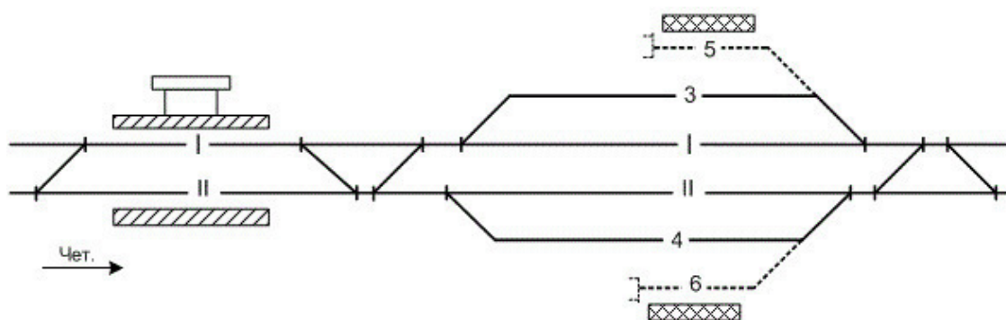
Рис. 2.3. Обгонный пункт
