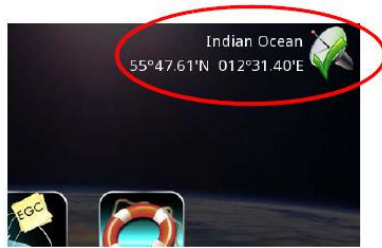
Рис. 3 Процедура Login
