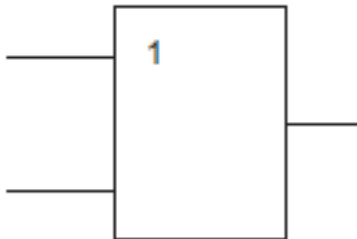
Рис. 1.3. Условное графическое обозначение логического элемента «ИЛИ»
