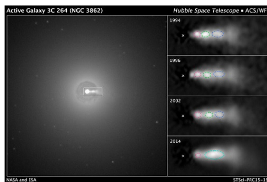
Рис.4 Компьютерная анимация процессов в джете
