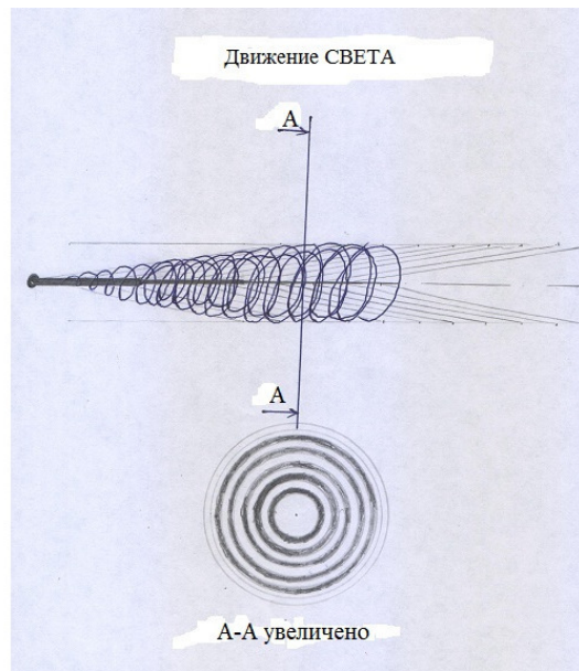
Рис.31 СВЕТОЭфирный поток
