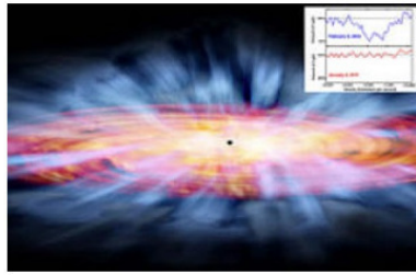
Рис.16 Квazar. Внутри чёрная точка-шаровая область из Света ничего не излучающая, поэтому кажущаяся чёрной, которую считают чёрной дырой
