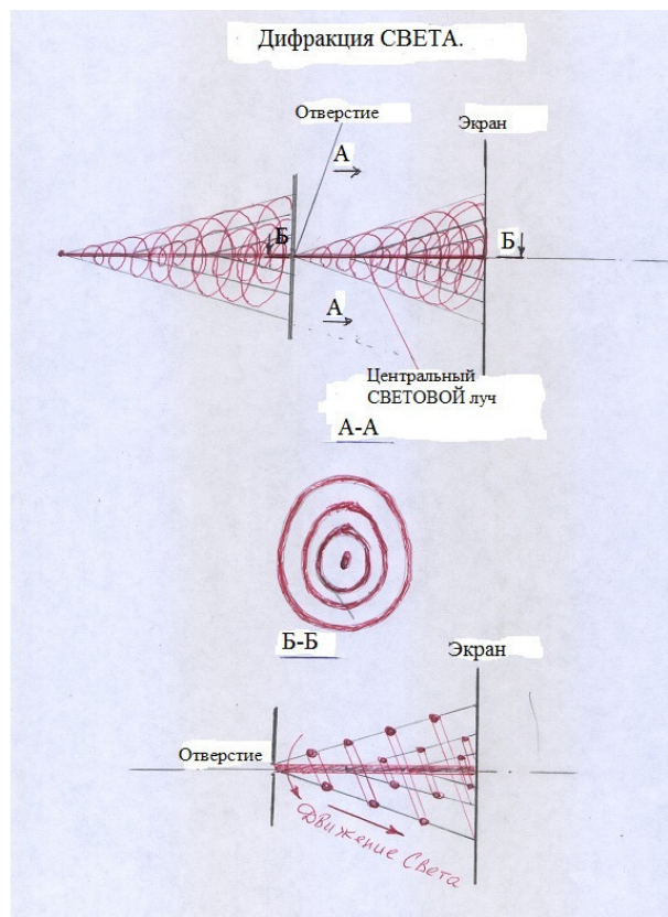
Рис.32 Дифракция СВЕТА
