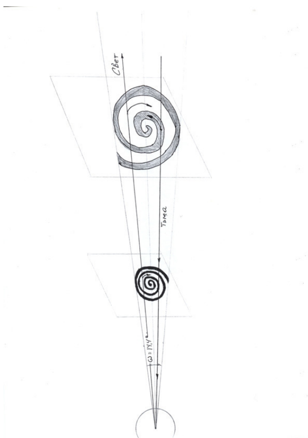
Рис.24 СВЕТОЭфирный поток
