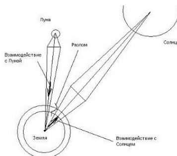
Рис. 23 Гравитационное взаимодействие Земли с Луной и Солнцем
