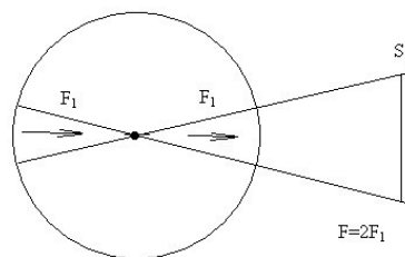
Рис. 22 Формирование силы гравитационного воздействия на тело
