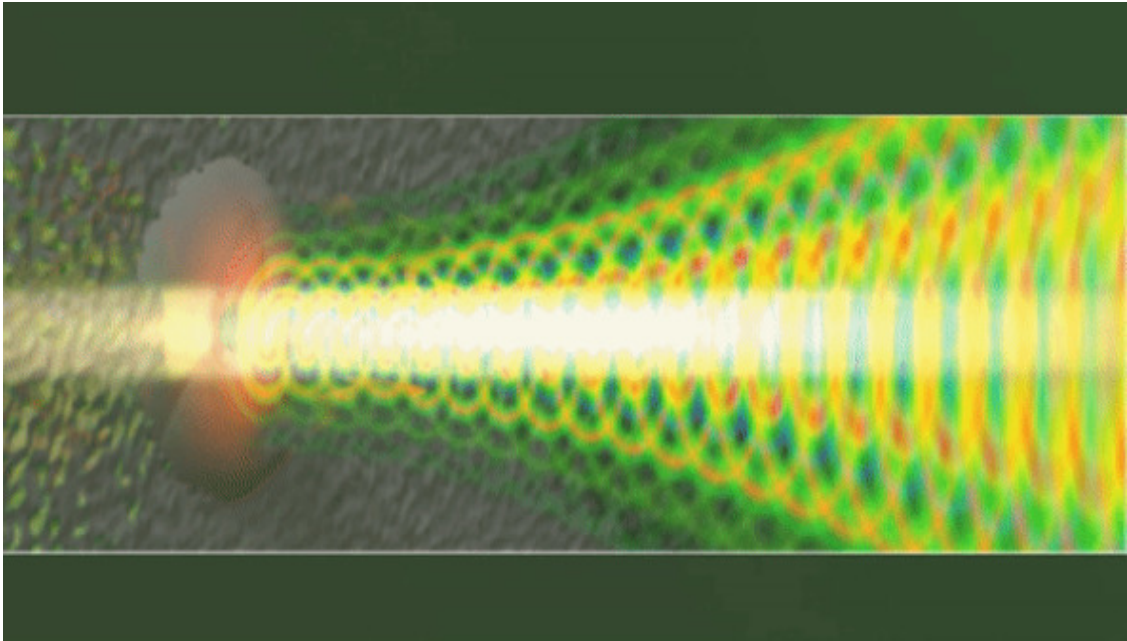
Рис.35 Схема образования наноиголки на поверхности металла под действием оптического вихря.
