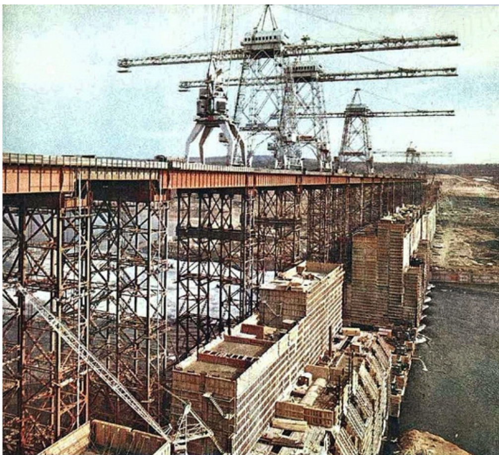
Строительство Усть-Илимской ГЭС
