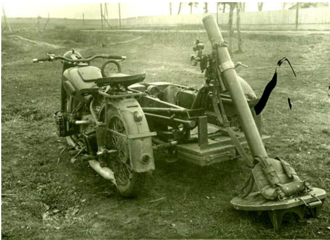
Миномёт приспособленный к мотоциклу
