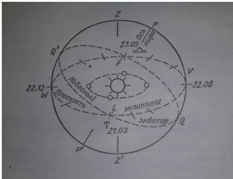
рис. 2. Видимое движение Солнца
