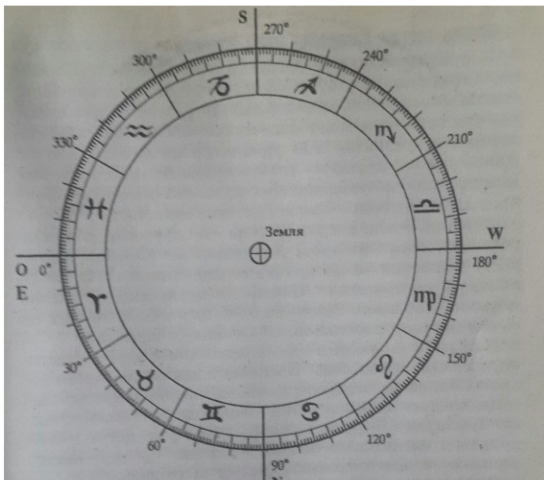
рис. 3. Зодиакальный круг
