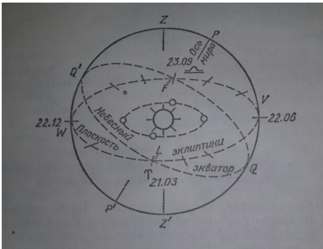
рис. 2. Видимое движение Солнца
