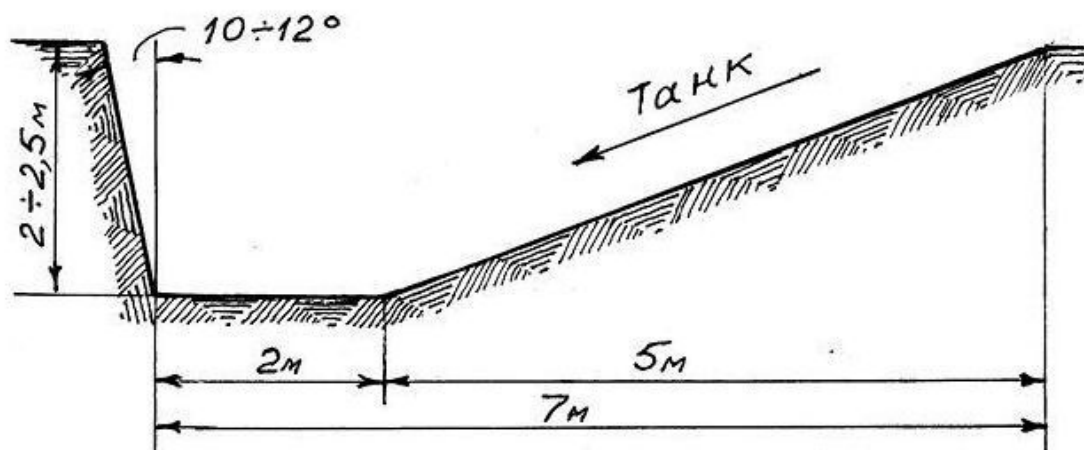
Рис. 1. Поперечный разрез противотанкового рва
