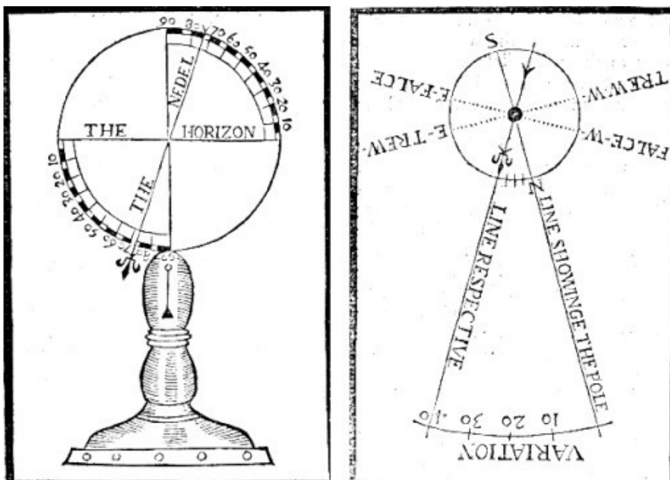
Рис 3. измеритель наклона Нормана и схема поясняющая его работу по [9].
