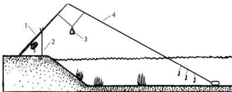
Рис. 2. Донка для весенней ловли голавля: 1 – спиннинг; 2 – подставка; 3 – сторожок-колокольчик (можно не использовать); 4 – основная леска.
