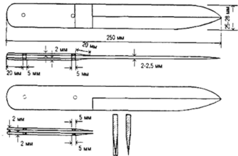
Рис. 2 Размеры Ножа
