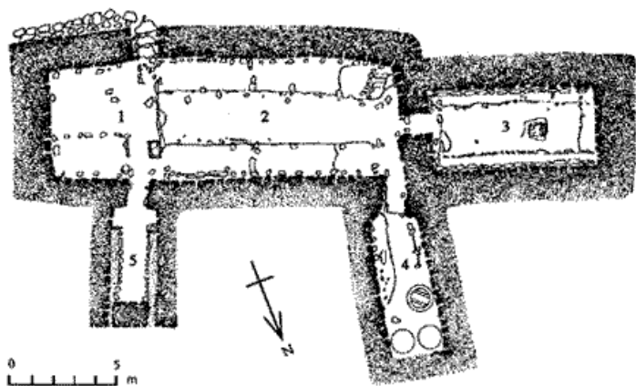
План исландского хутора периода викингов (по материалам раскопок): 1 – сени; 2 – центральное жилое помещение («зал»); 3 – рабочая комната; 4 – чулан; 5 – уборная
